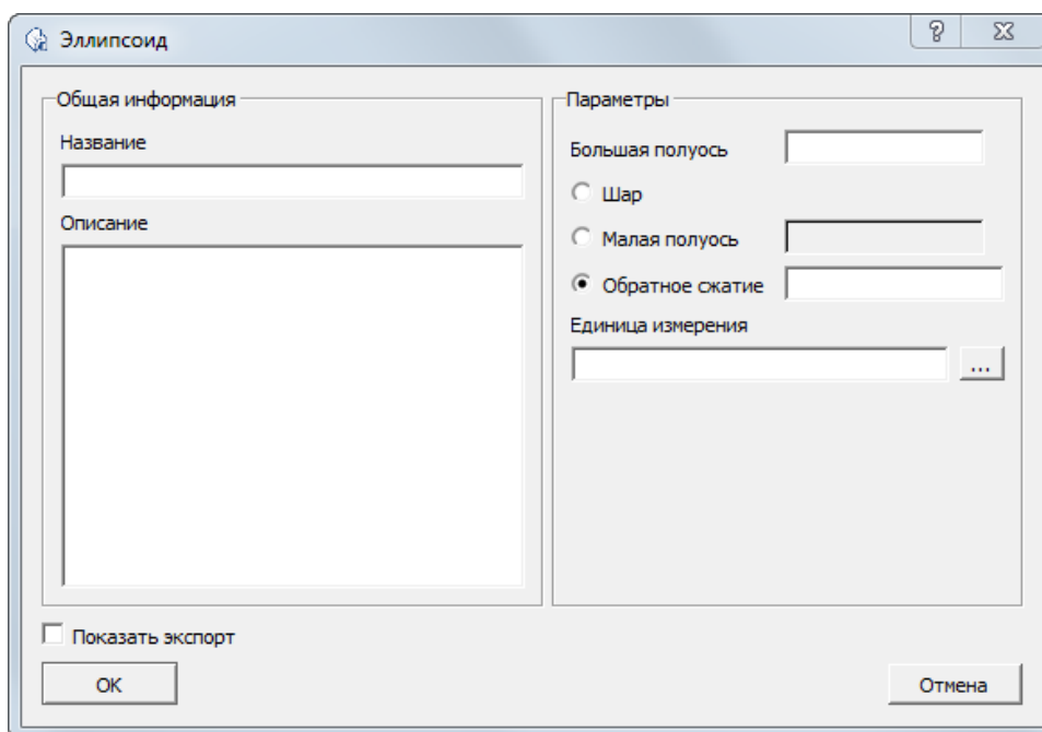
Рис. 26. Параметры референц-эллипсоида
