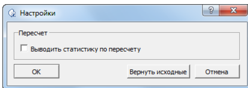
Рис. 2. Настройки программы
