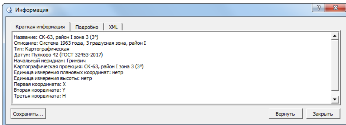
Рис. 5. Окно «Информация»
