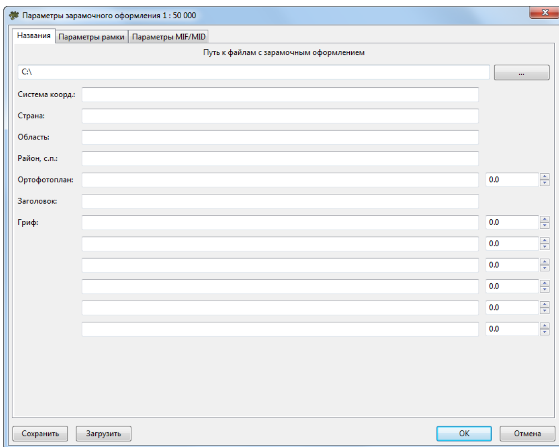
Рис. Б.30. Параметры зарамочного оформления ортофотоплана для системы MapInfo в условных знаках масштаба 1:50 000, закладка «Названия»
