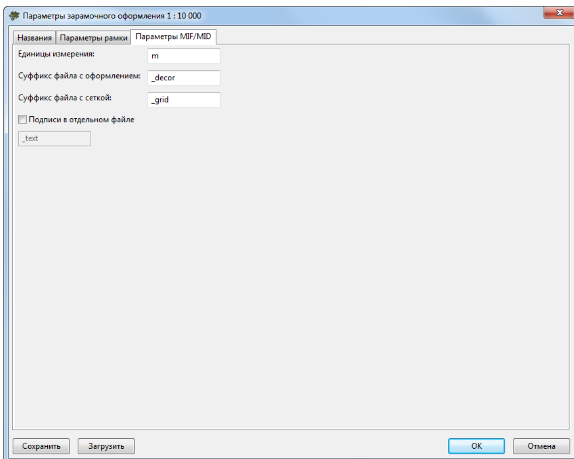
Рис. Б.20. Параметры автоматического оформления ортофотоплана для системы MapInfo в условных знаках масштаба 1:10 000, закладка «Параметры MIF/MID»
