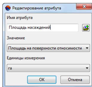
Рис. 16. Редактирование атрибута
