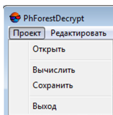
Рис. 29. Меню «Проект»
