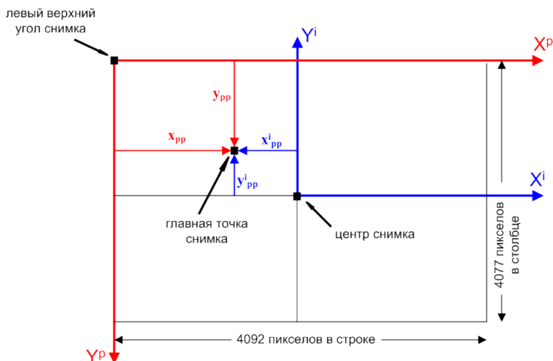
Рис. 17. Связь систем координат снимка и монитора
