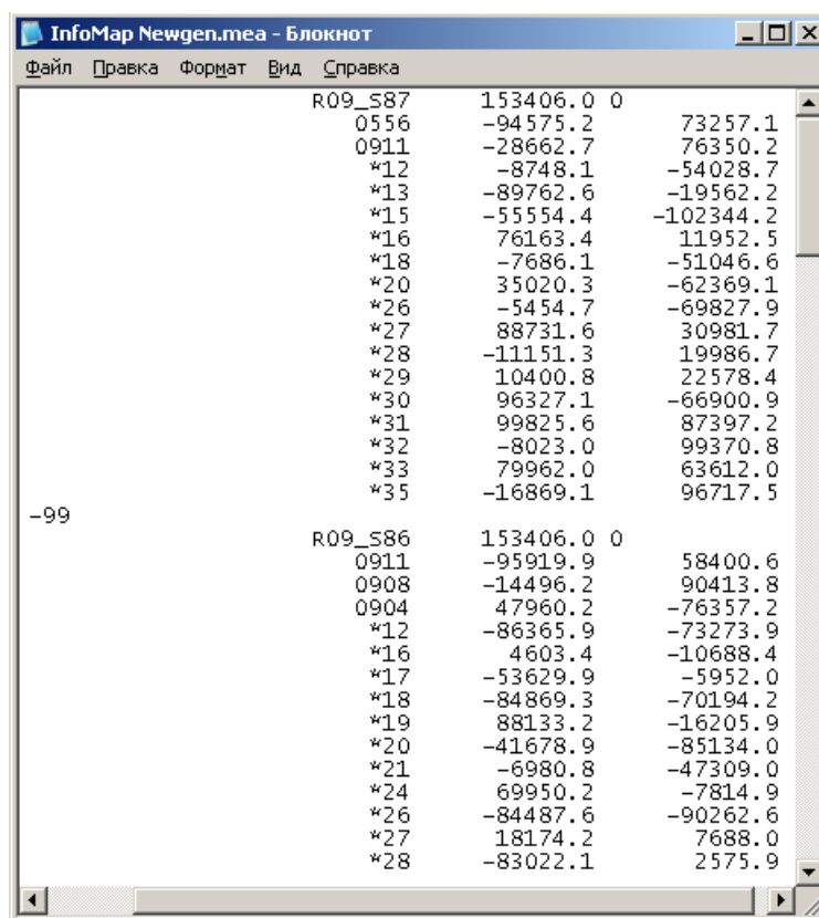
Рис. 144. Пример файла измерений координат точек на снимках
