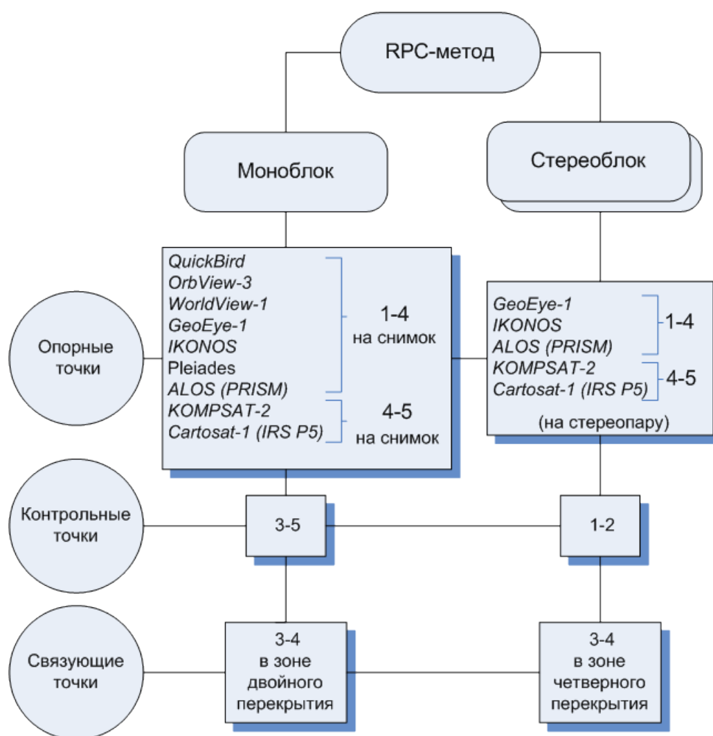
Рис. 146. Количество точек, рекомендуемое для уравнивания сканерного блока с использованием RPC
