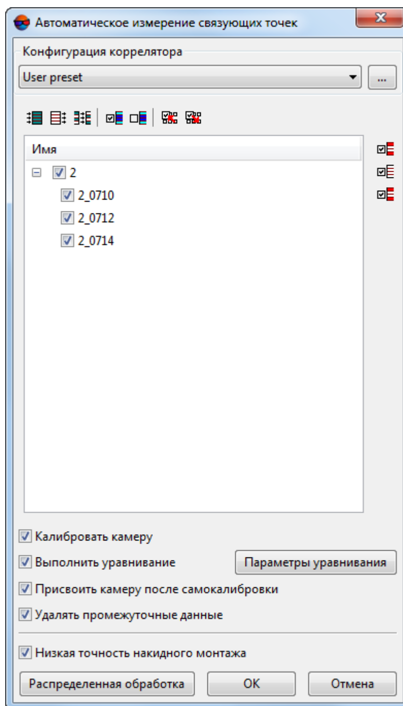
Рис. 62. Окно «Автоматическое измерение связующих точек»
