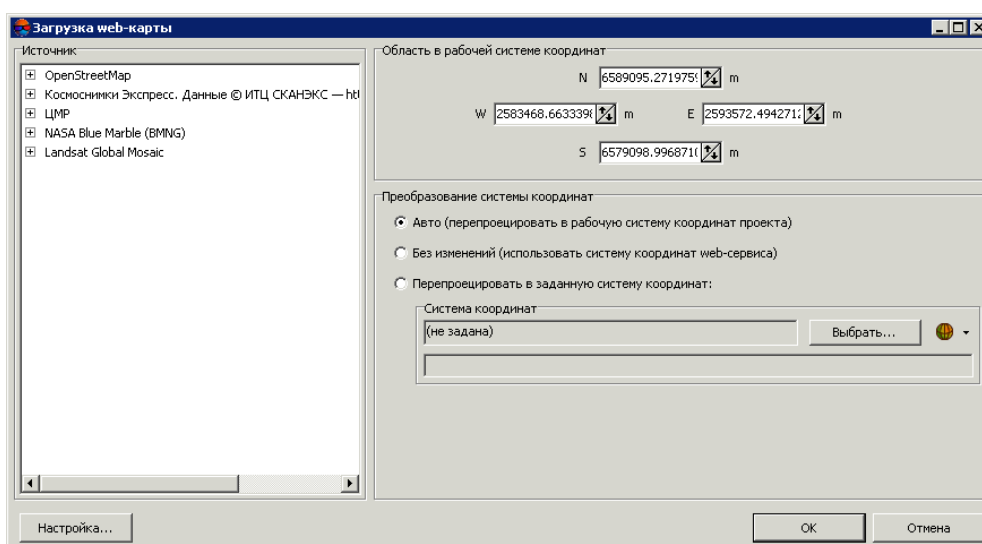
Рис. 107. Параметры загрузки web-карты
