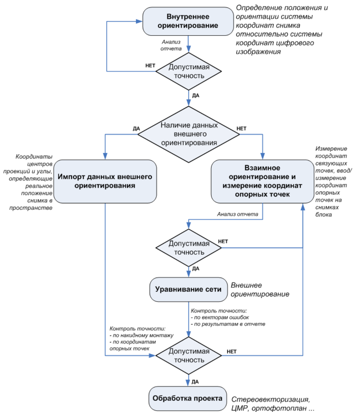
Рис. 1. Схема действий при построении сети фототриангуляции
