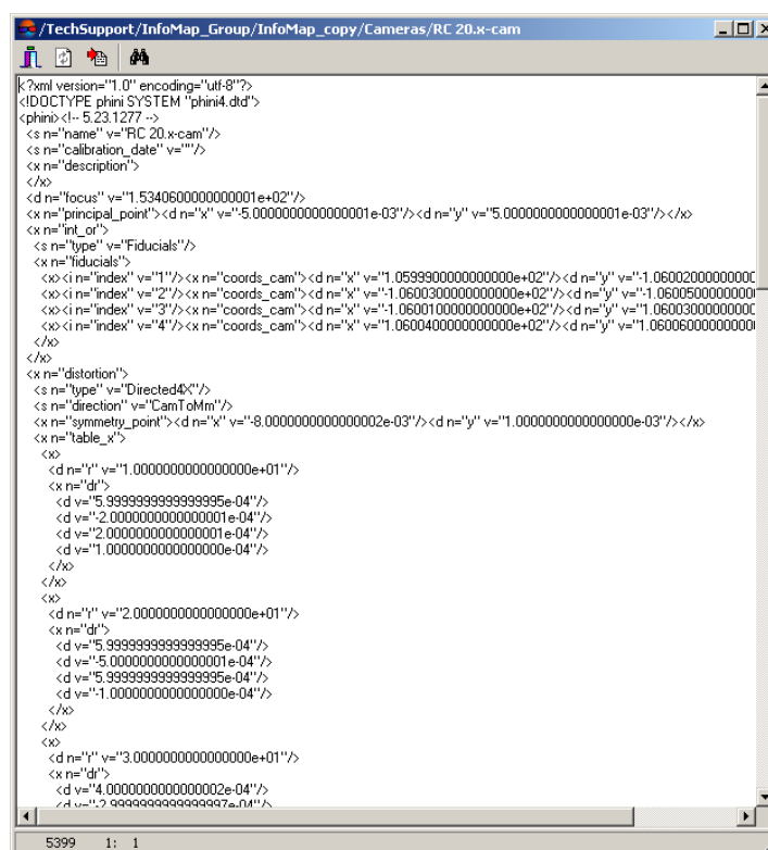
Рис. 22. Параметры камеры в файле формата *.x-cam
