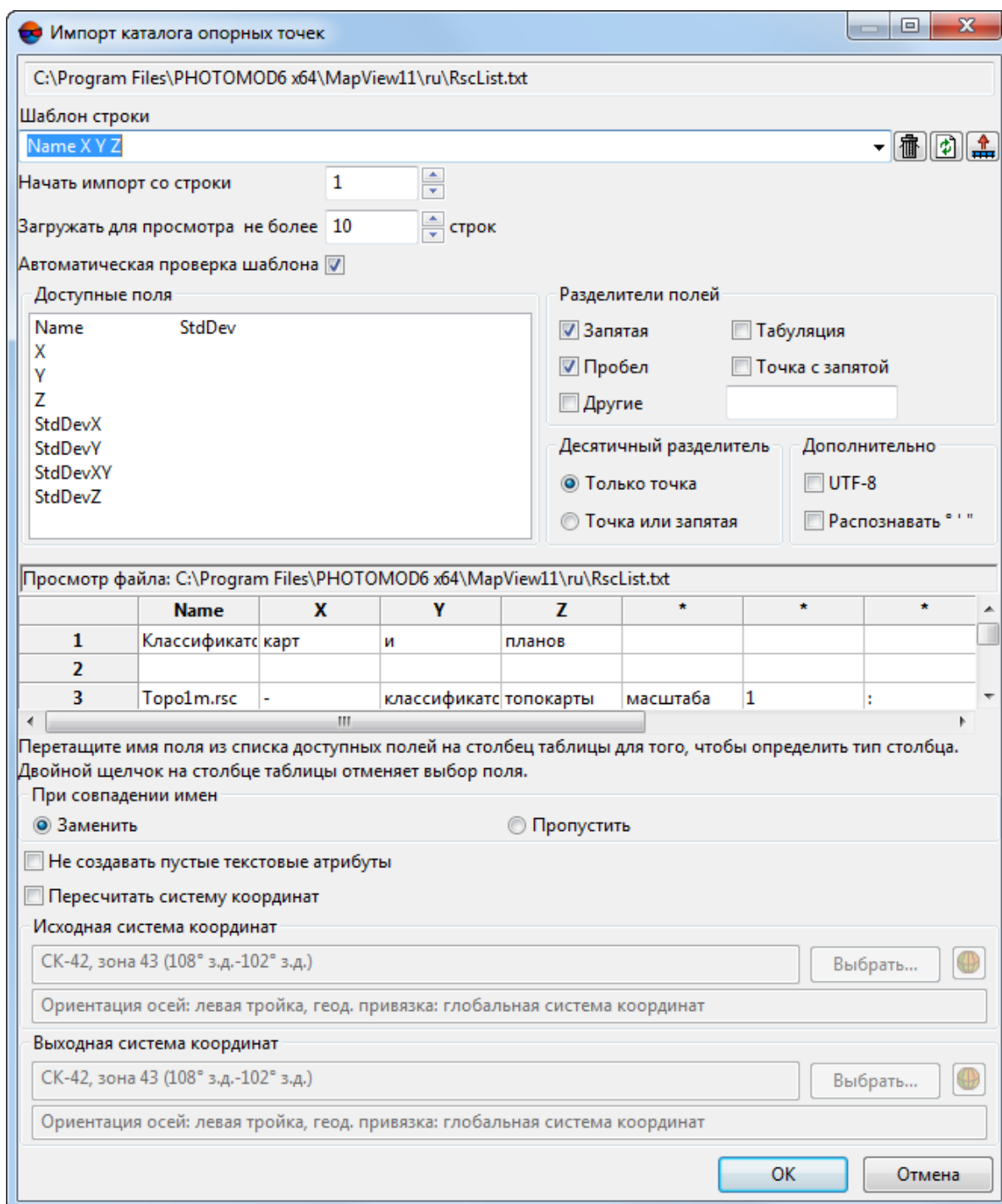
Рис. 96. Импорт каталога опорных точек
