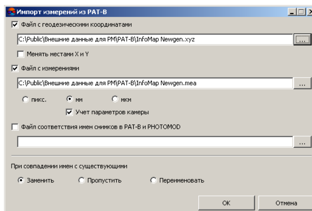
Рис. 130. Импорт измерений из PAT-B
