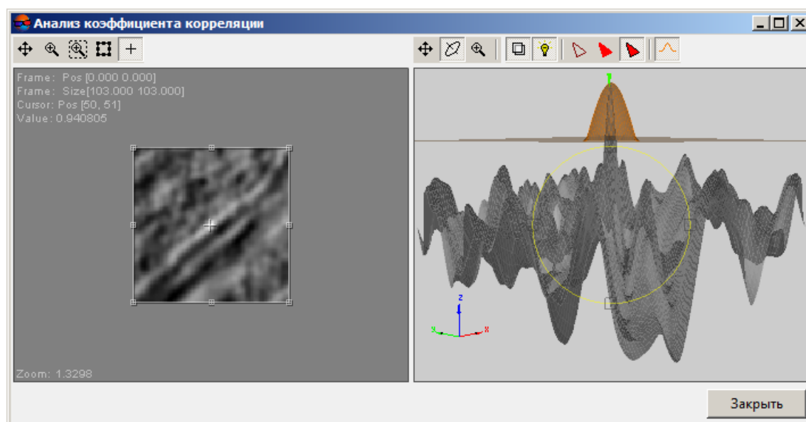
Рис. 78. Анализ коэффициента корреляции
