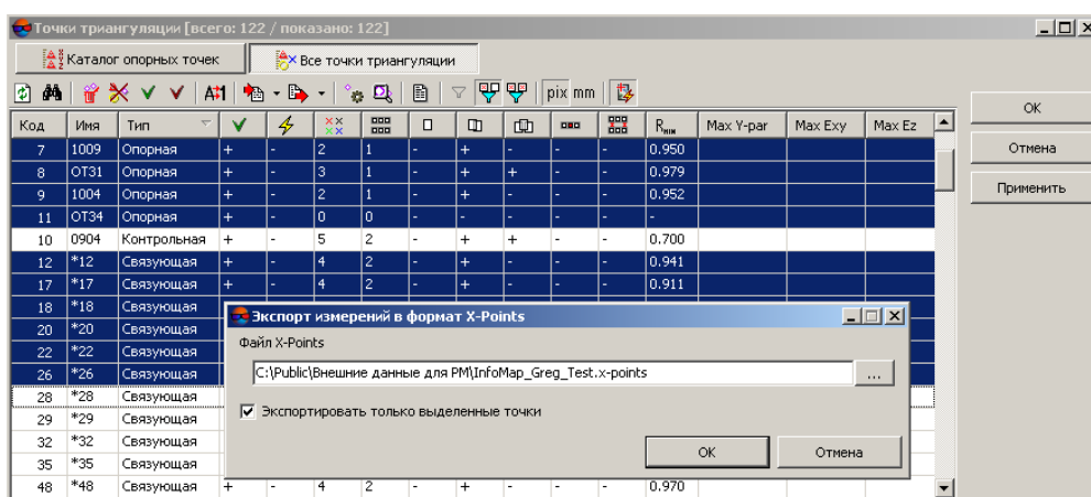
Рис. 137. Экспорт выделенных точек триангуляции в файл формата X-Points
