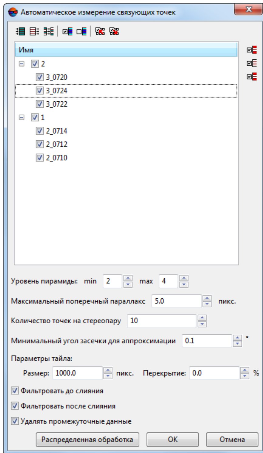
Рис. 53. Окно «Автоматическое измерение связующих точек»
