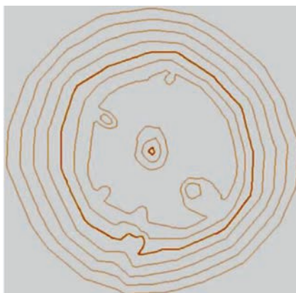
Рис. 7. Построение горизонталей по матрице высот и формирование среза грунта
