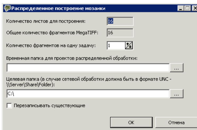
Рис. 62. Параметры распределенного построения мозаики
