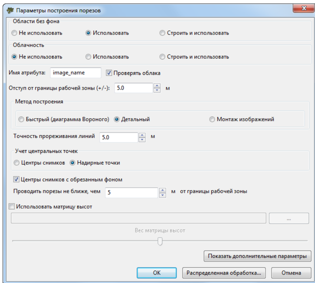
Рис. 18. Параметры построения порезов в автоматическом режиме
