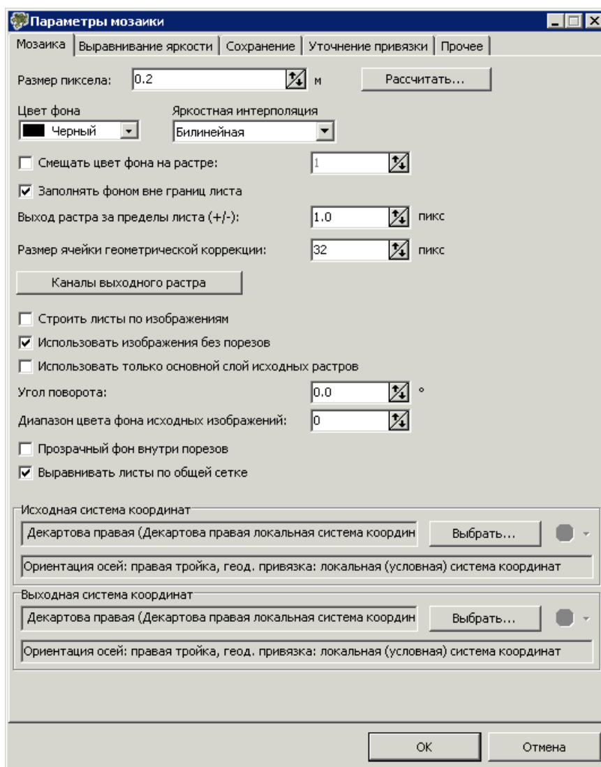
Рис. 56. Окно «Параметры мозаики»
