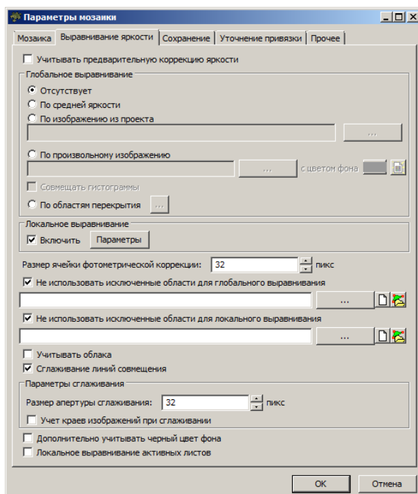
Рис. 24. Параметры выравнивания яркости
