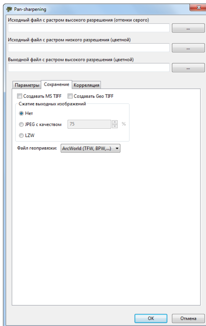
Рис. 73. Закладка Сохранение окна Pan-sharpening
