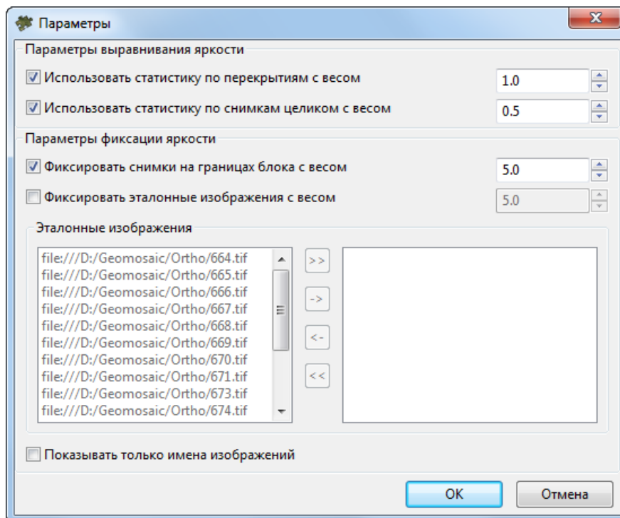
Рис. 25. Параметры выравнивания яркости по областям перекрытия
