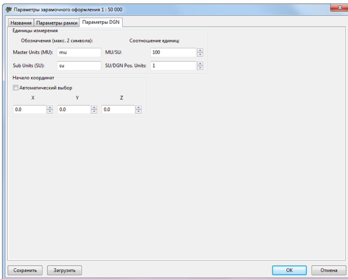
Рис. 108. Параметры зарамочного оформления ортофотоплана для системы MicroStation в условных знаках масштаба 1:50 000, закладка «Параметры DGN»
