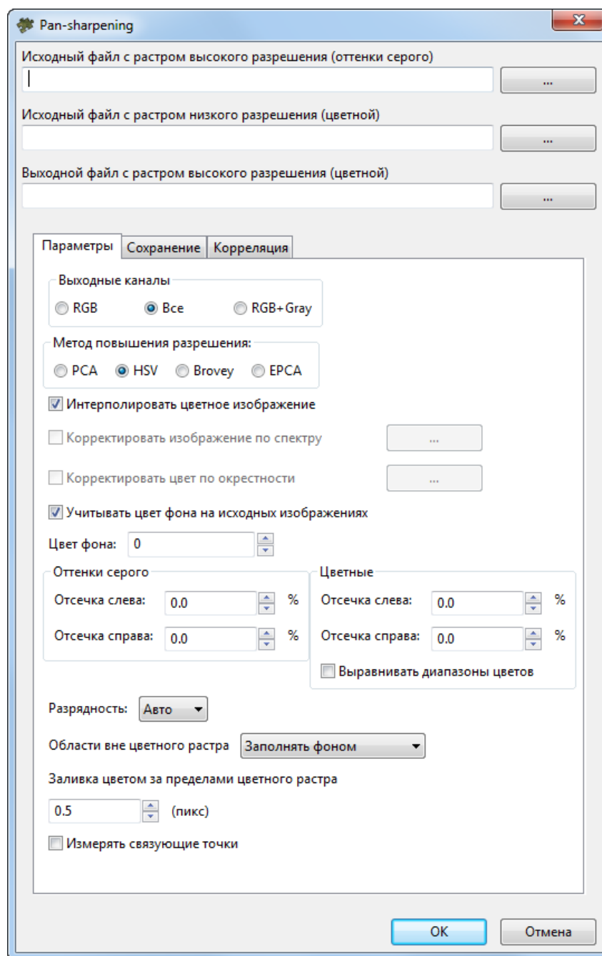
Рис. 63. Окно настройки операции Pan-sharpening
