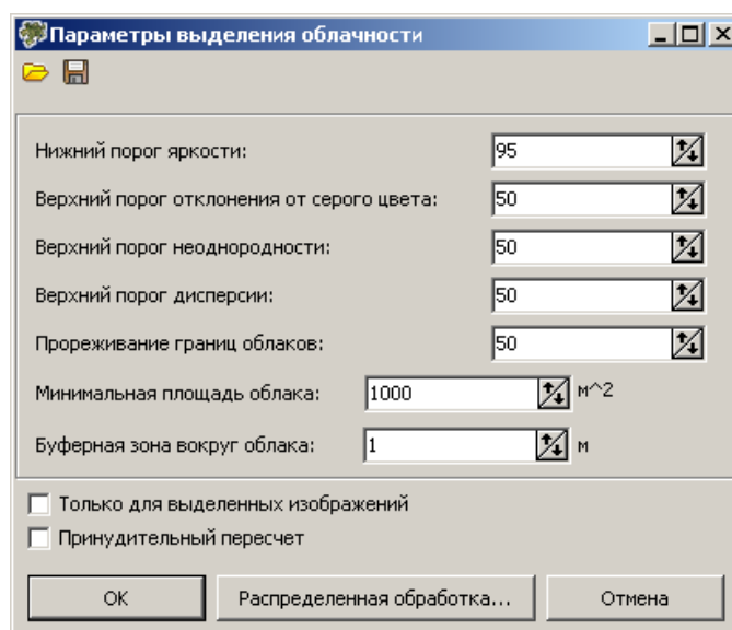
Рис. 16. Параметры выделения облачности
