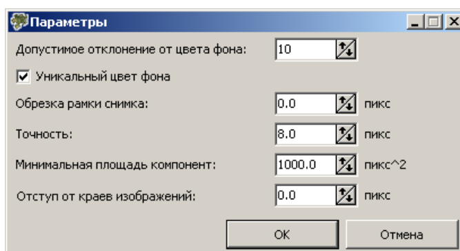
Рис. 51. Параметры построения полигонов по границам изображений без учета фона
