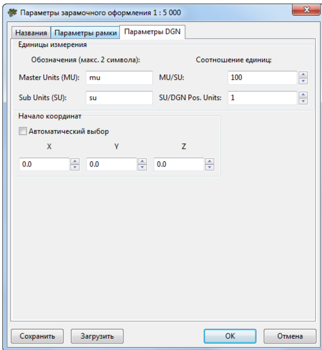
Рис. 90. Параметры зарамочного оформления ортофотоплана для системы MicroStation в условных знаках масштаба 1:5 000, закладка «Параметры DGN»
