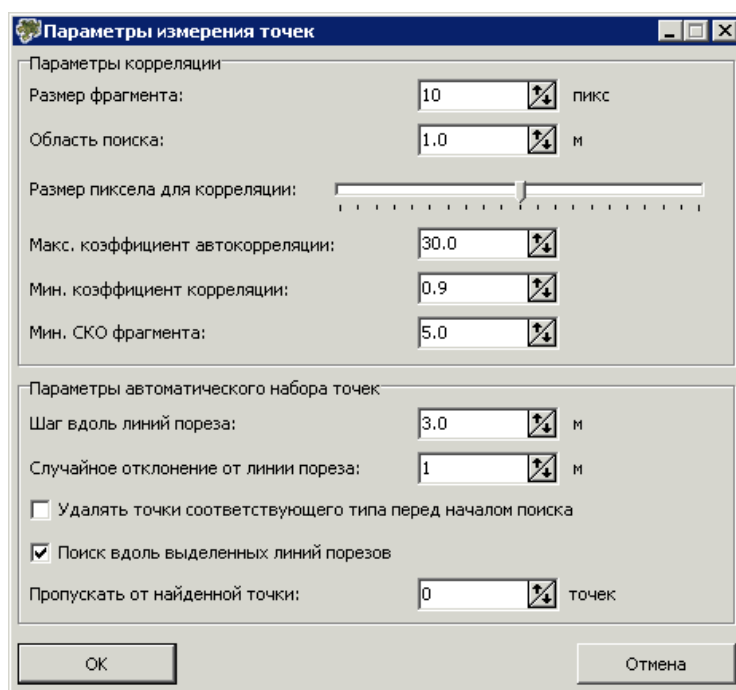
Рис. 37. Параметры измерения точек
