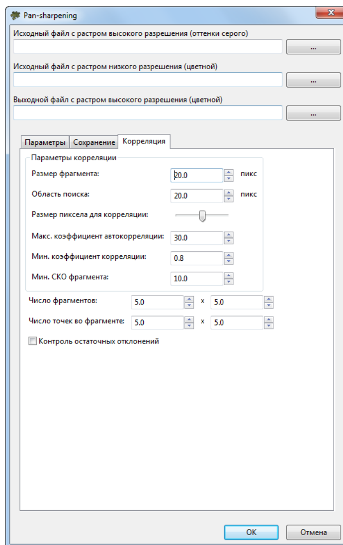
Рис. 74. Закладка Корреляция окна Pan-sharpening
