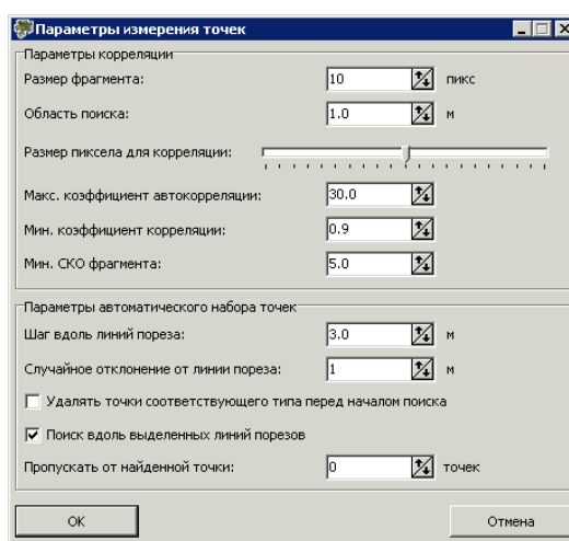
Рис. 32. Параметры измерения точек
