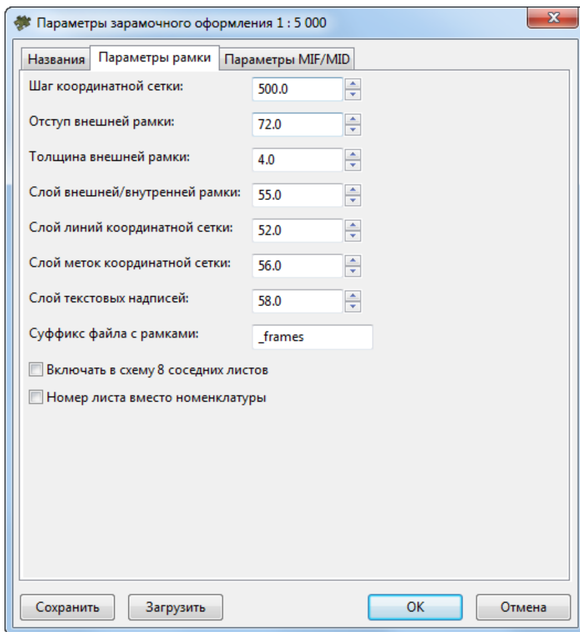
Рис. 92. Параметры зарамочного оформления ортофотоплана для системы MapInfo в условных знаках масштаба 1:5 000, закладка «Параметры рамки»
