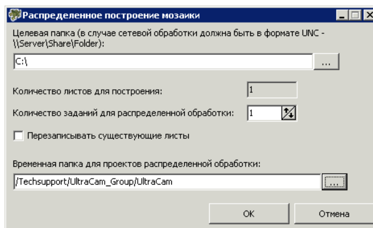
Рис. 61. Параметры распределенного построения мозаики
