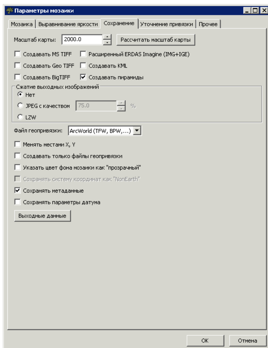
Рис. 58. Параметры сохранения мозаики
