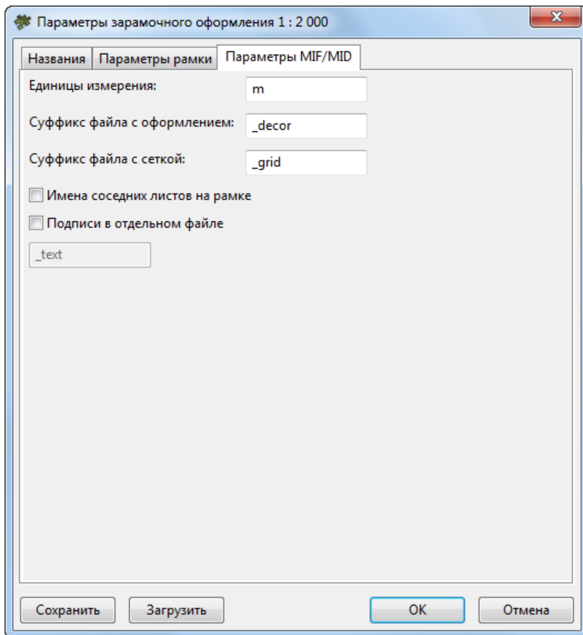
Рис. 87. Параметрыaramочного оформления ортофотоплана для системы MapInfo в условных знаках масштаба 1:2 000, закладка «Параметры MIF/MID»
