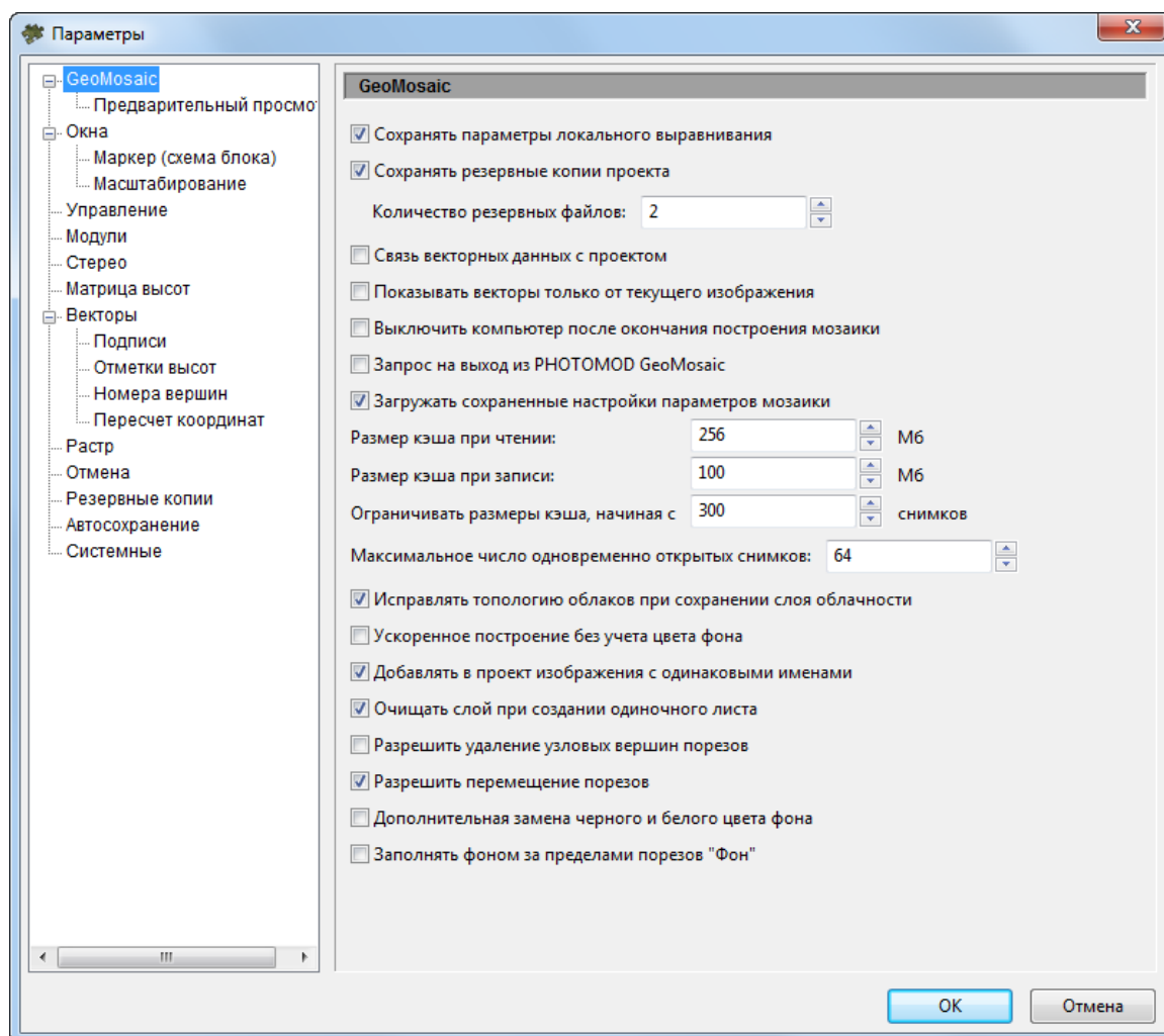
Рис. 78. Общие параметры программы
