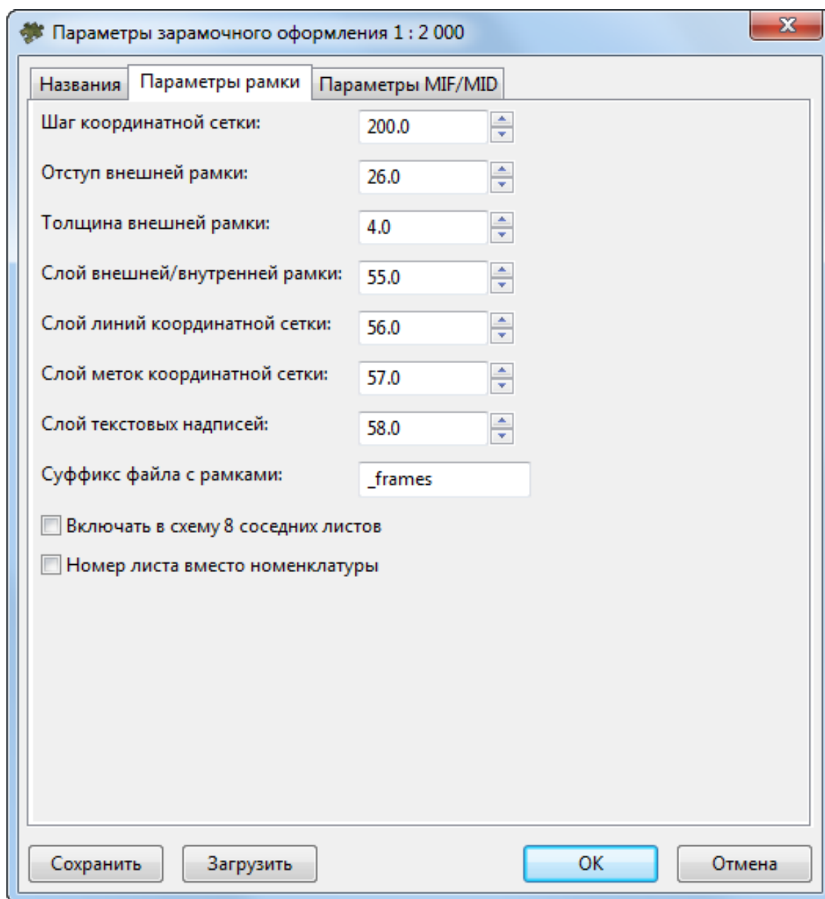
Рис. 86. Параметры зарамочного оформления ортофотоплана для системы MapInfo в условных знаках масштаба 1:2 000, закладка «Параметры рамки»
