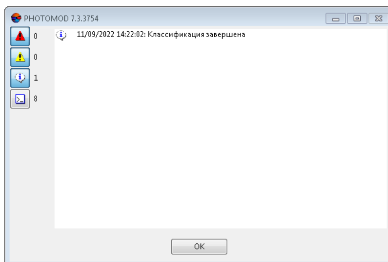
Рис. 31. Информационное сообщение
