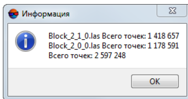
Рис. 2. Окно «Информация»
