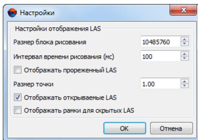
Рис. 3. Окно «Настройки»
