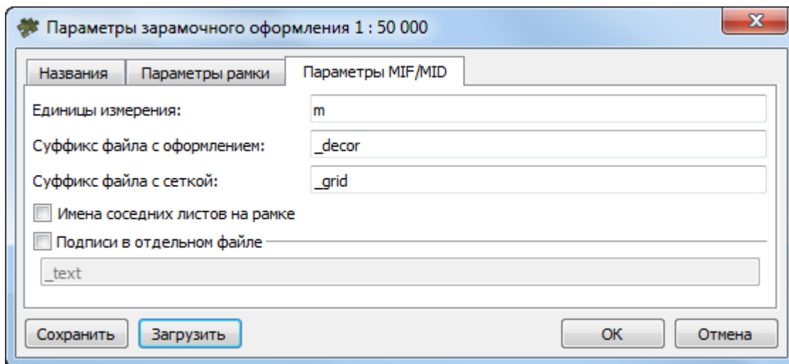
Рис. В.32. Параметры зарамочного оформления ортофотоплана для системы MapInfo в условных знаках масштаба 1:50 000, закладка «Параметры MIF/MID»
