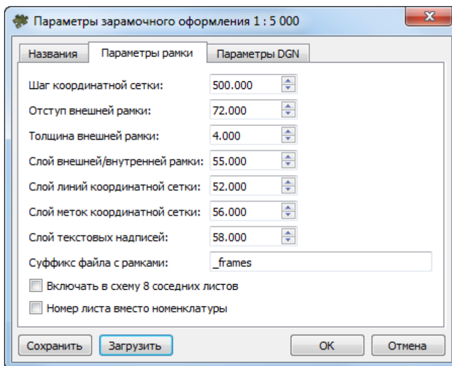
Рис. В.10. Параметры зарамочного оформления ортофотоплана для системы MicroStation в условных знаках масштаба 1:5 000, закладка «Параметры рамки»
