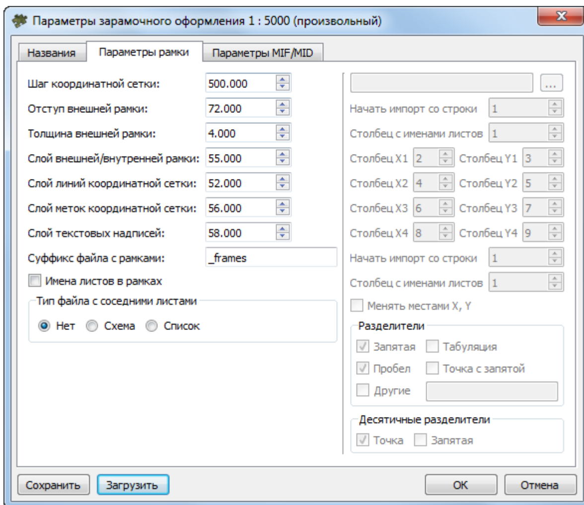
Рис. В.34. Закладка «Параметры рамки» окна с расширенными возможностями редактирования зарамочного оформления для системы MapInfo в условных знаках масштаба 1:5 000
