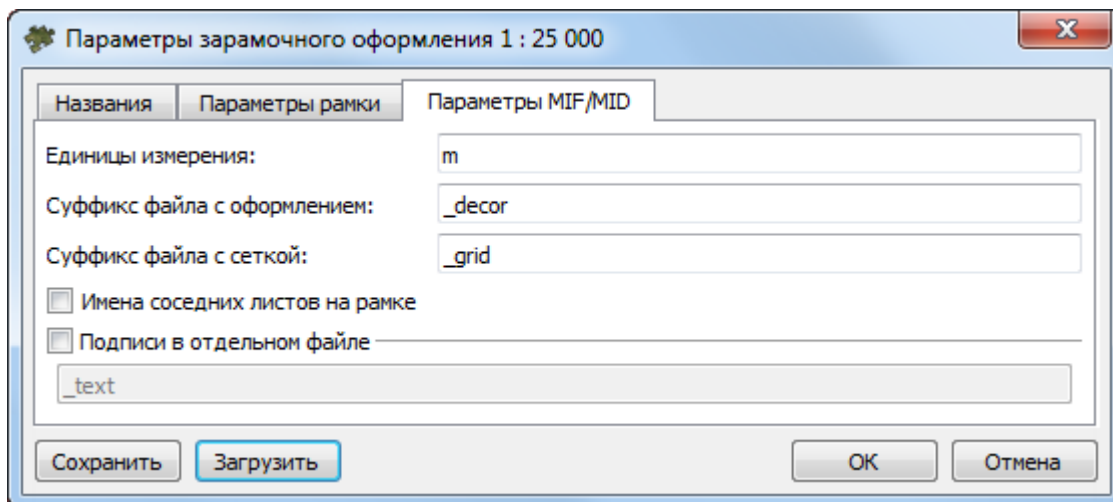
Рис. В.26. Параметры зарамочного оформления ортофотоплана для системы MapInfo в условных знаках масштаба 1:25 000, закладка «Параметры MIF/MID»
