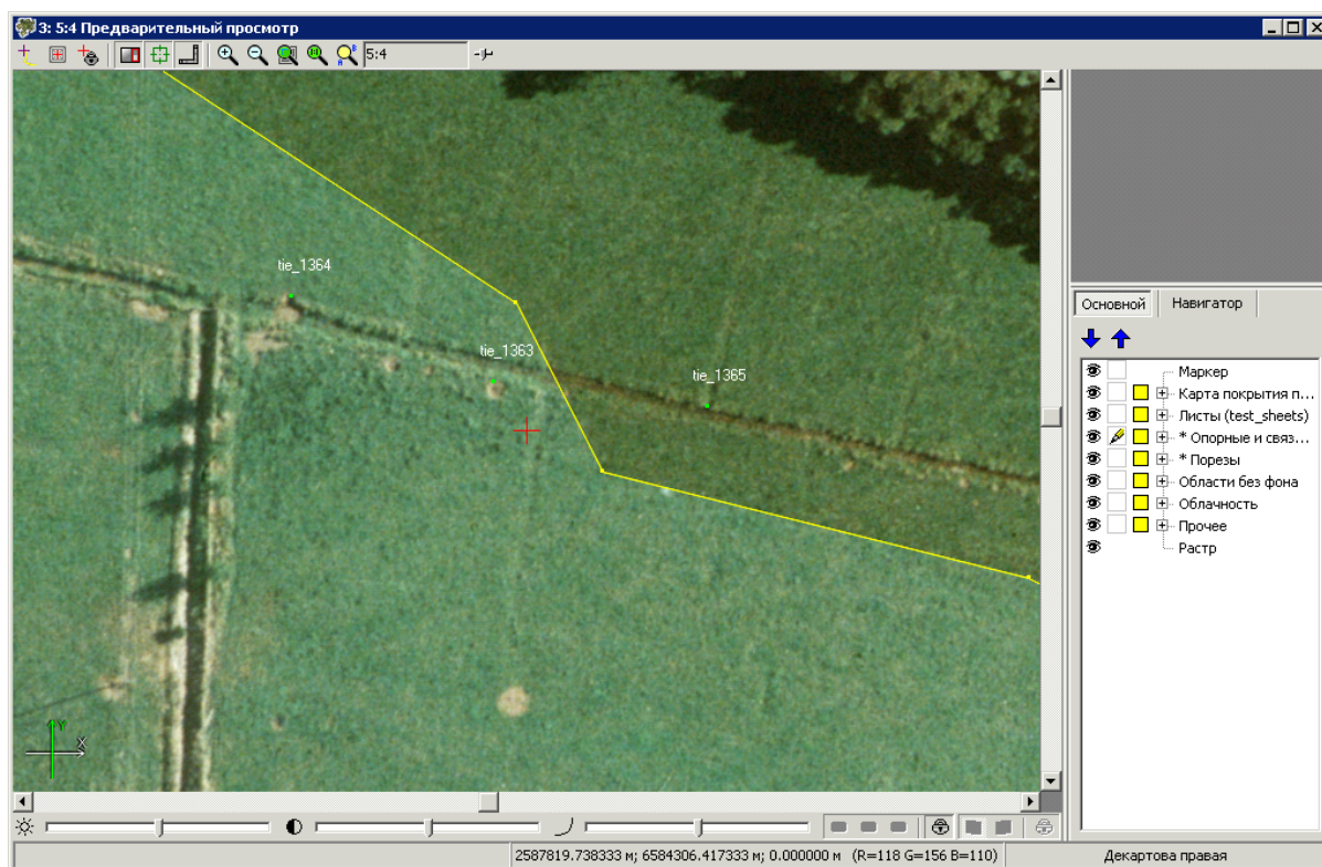
Рис. 42. Сшивка областей по двум связующим точкам
