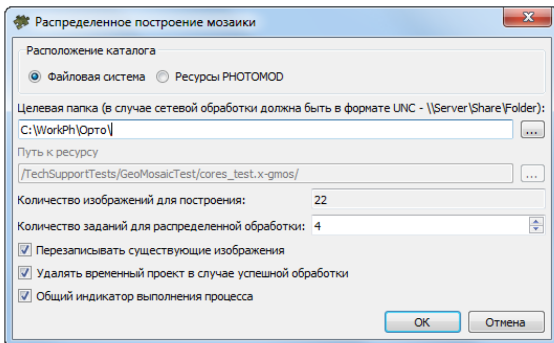
Рис. 73. Параметры распределенного построения мозаики
