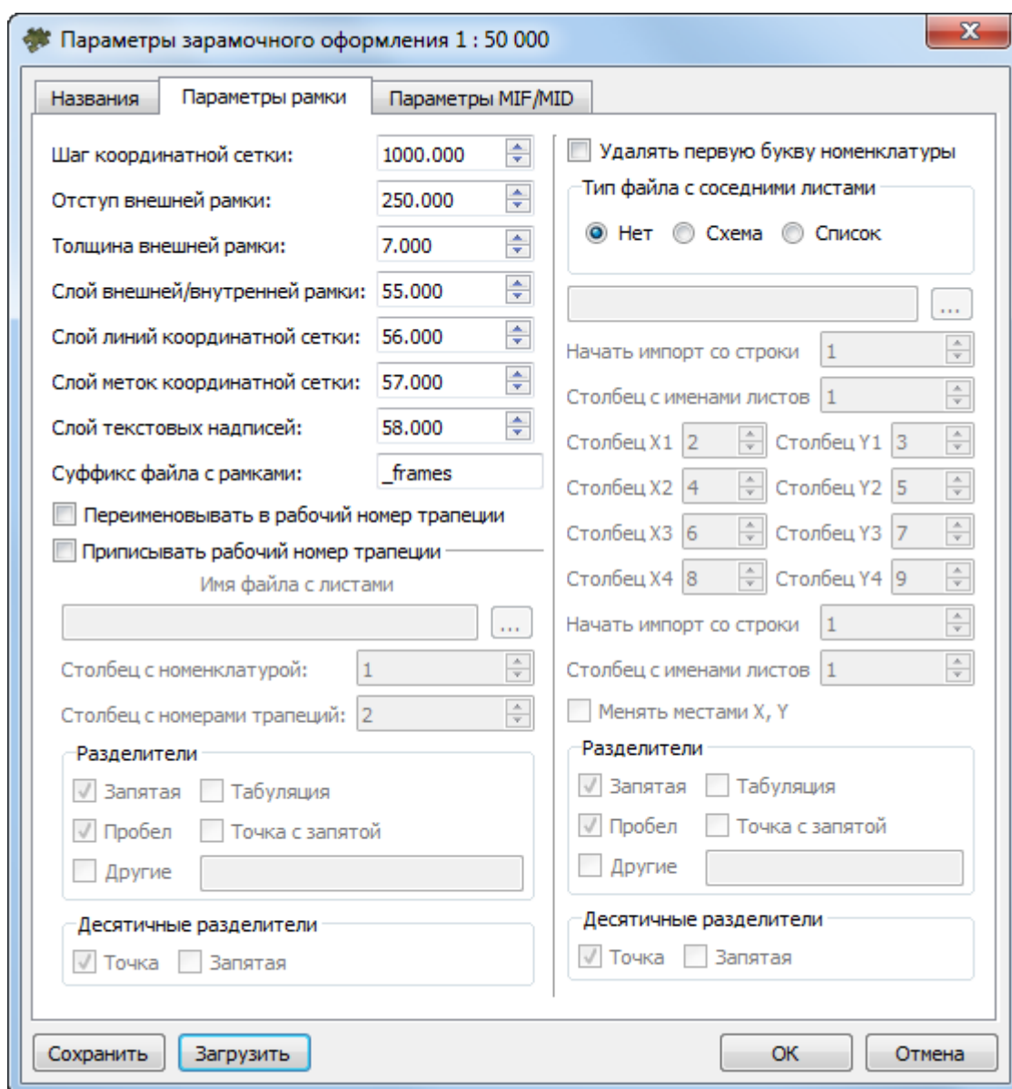
Рис. В.31. Параметры зарамочного оформления ортофотоплана для системы MapInfo в условных знаках масштаба 1:50 000, закладка «Параметры рамки»
