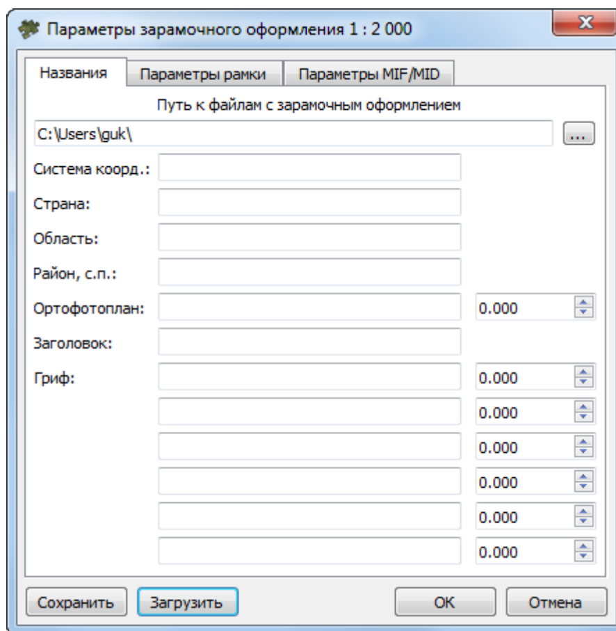
Рис. В.6. Параметры зарамочного оформления ортофотоплана для системы MapInfo в условных знаках масштаба 1:2 000, закладка «Названия»
