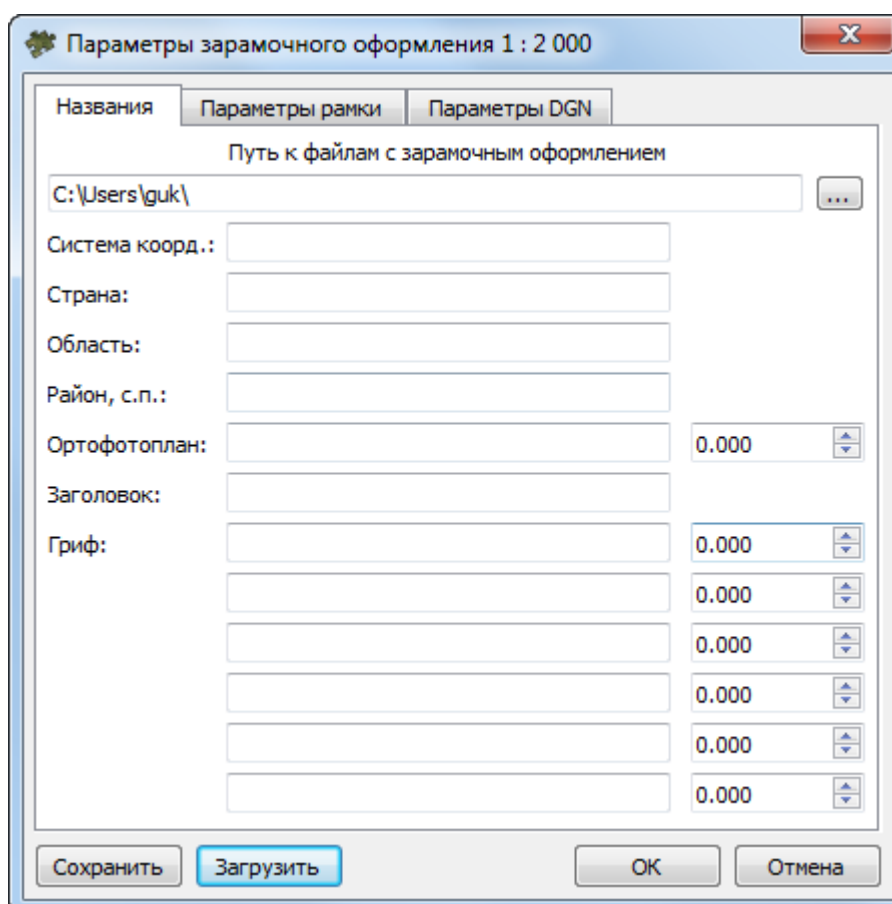
Рис. В.3. Параметры зарамочного оформления ортофотоплана для системы MicroStation в условных знаках масштаба 1:2 000, закладка «Названия», пример заполнения
