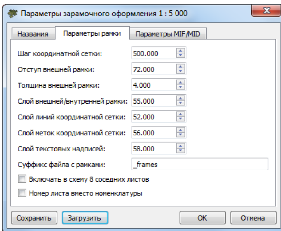
Рис. В.13. Параметры зарамочного оформления ортофотоплана для системы MapInfo в условных знаках масштаба 1:5 000, закладка «Параметры рамки»
