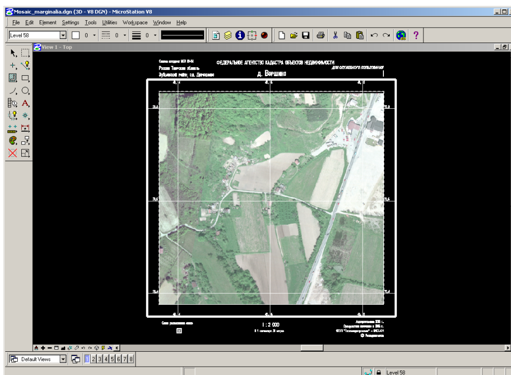
Рис. В.2. Ортофотоплан с зарамочным оформлением в окне программы MicroStation
