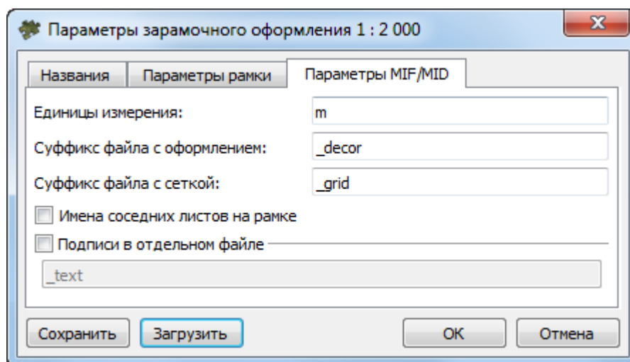
Рис. В.8. Параметры зарамочного оформления ортофотоплана для системы MapInfo в условных знаках масштаба 1:2 000, закладка «Параметры MIF/MID»
