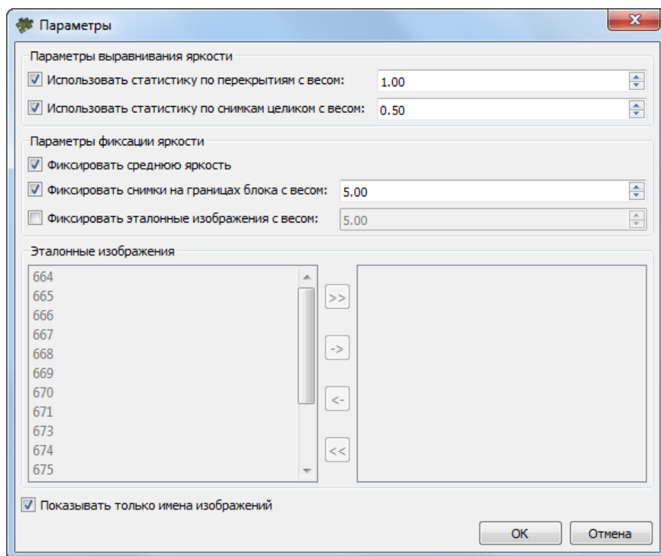
Рис. 32. Параметры выравнивания яркости по областям перекрытия
