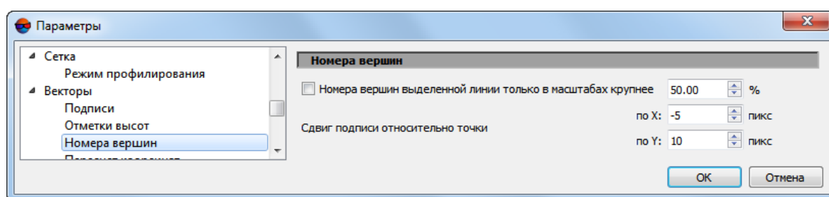
Рис. 18. Настройки отображения вершин выделенного векторного объекта
