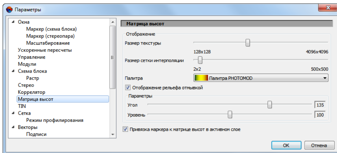
Рис. 11. Настройки отображения матрицы высот
