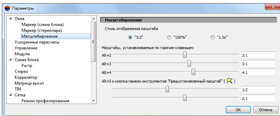
Рис. 3. Настройки масштабирования
