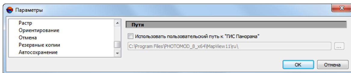
Рис. 28. Настройки путей
