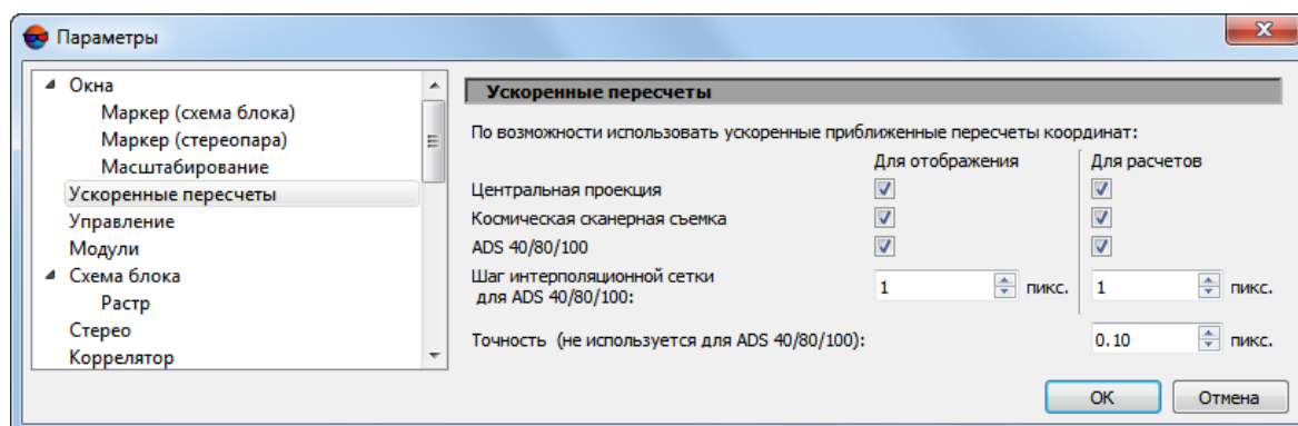
Рис. 4. Параметры быстрогодействия (для проекта ADS)
