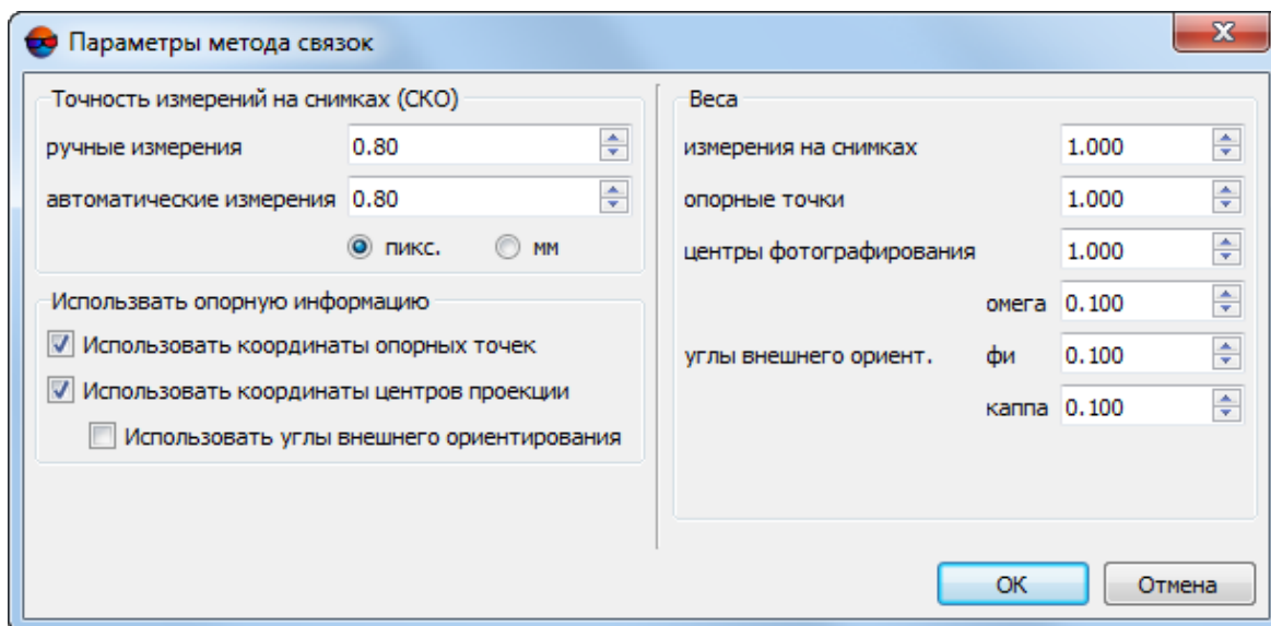
Рис. 16. Окно «Параметры метода связей»
