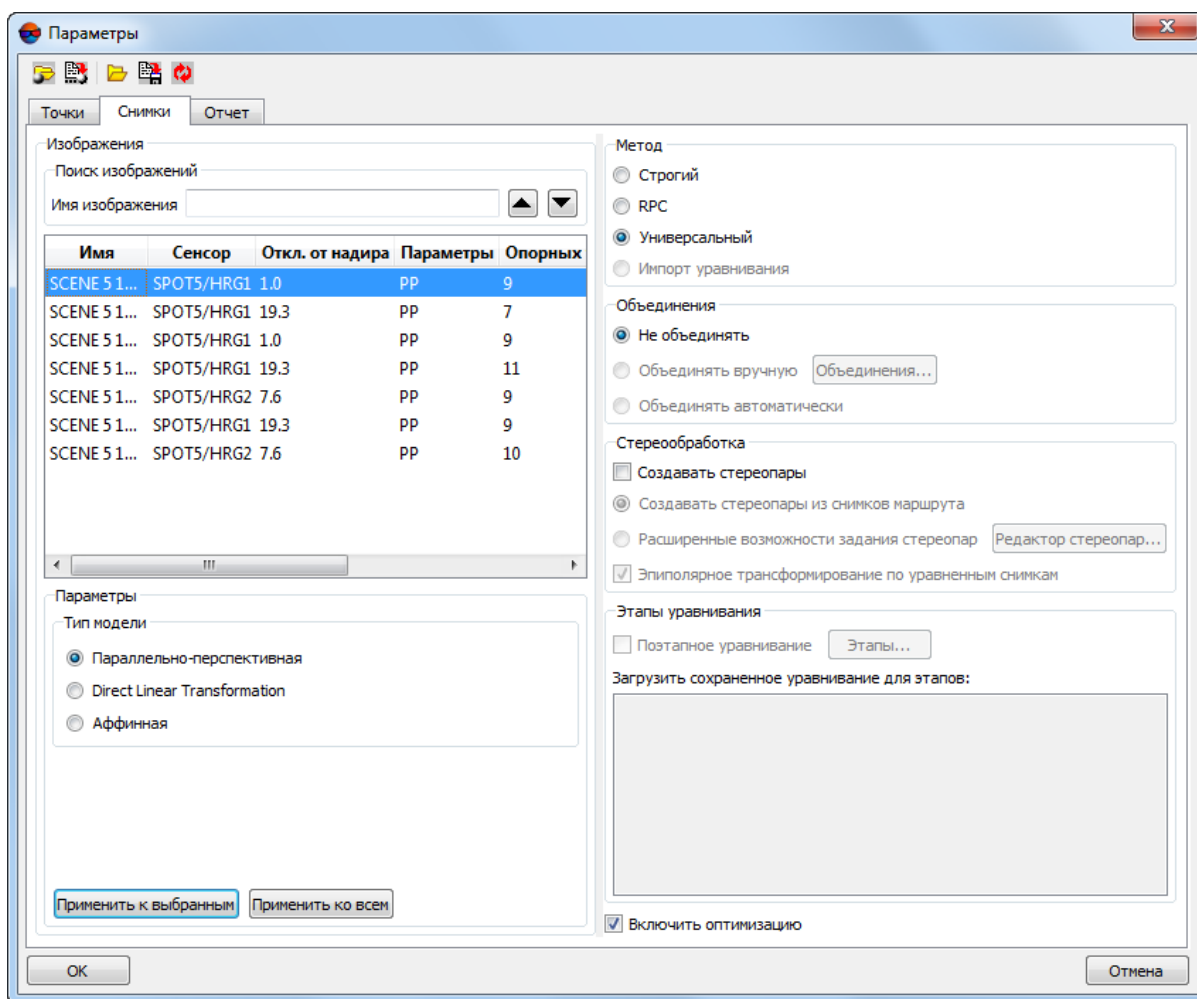
Рис. 29. Параметры универсального метода уравнивания снимков
