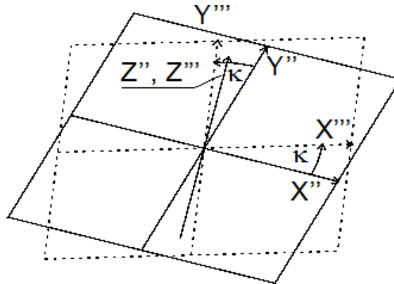
Рис. А.3. Положительный поворот вокруг оси Z на угол «каппа»
