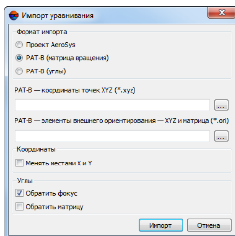
Рис. 48. Параметры импорта из проекта AeroSys
