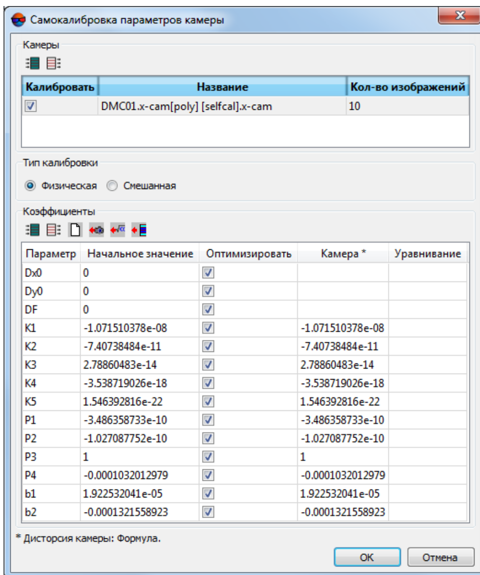
Рис. 17. Окно «Самокалибровка параметров камеры»
