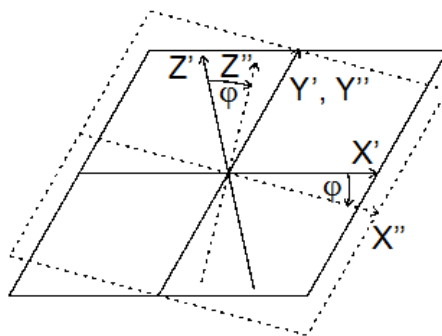
Рис. А.2. Положительный поворот вокруг оси Y на угол «фи»
