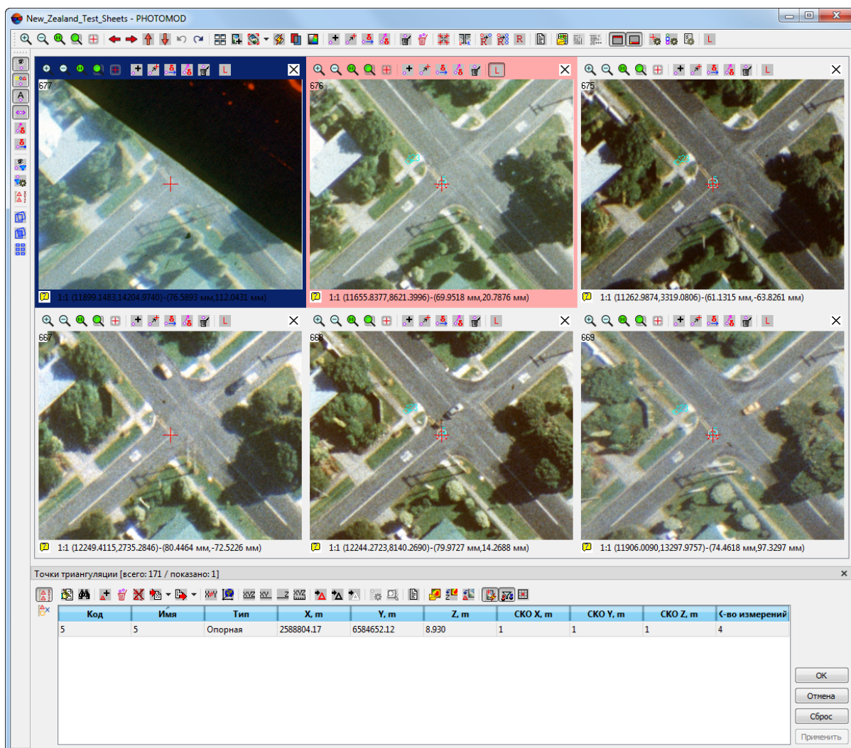
Рис. 46. Редактирование точек по списку
