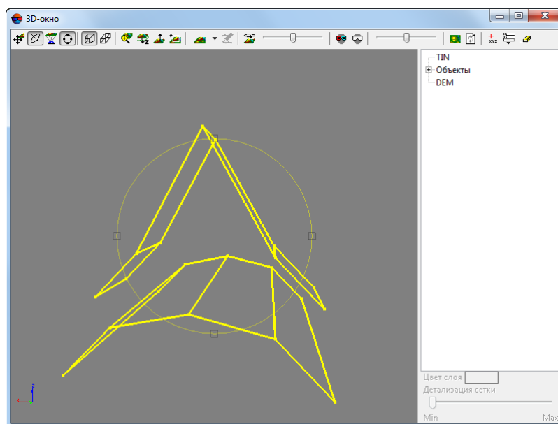
Рис. 53. Парапет над крышей типа «двускатная мансарда» в 3D-окне. Смещение по Z вершин парапета, расположенных над коньком крыши, увеличено вручную.
