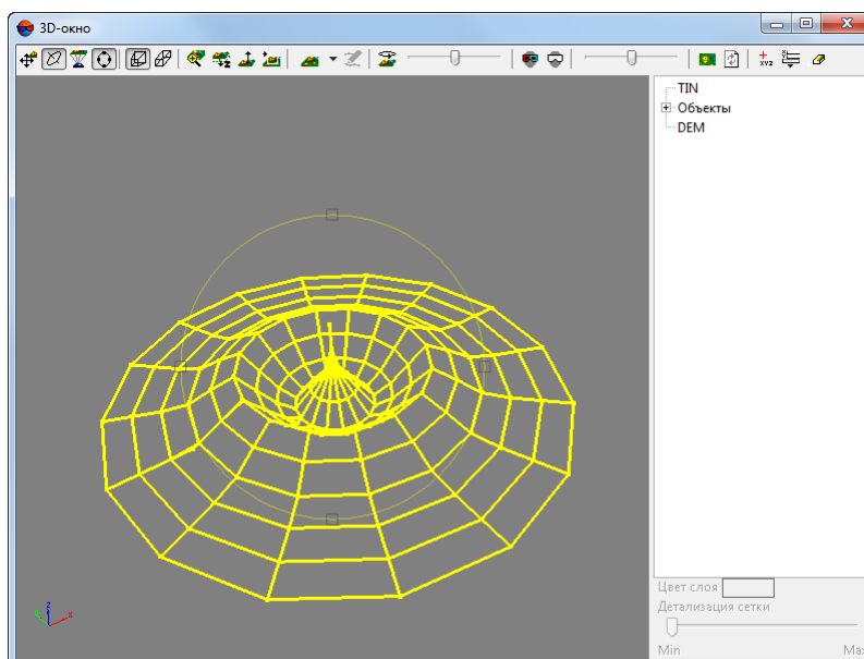
Рис. 61. Купол сложной формы, созданный вручную
