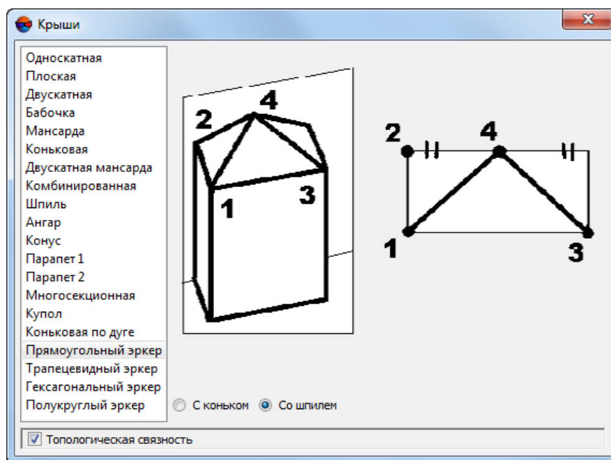
Рис. 64. Прямоугольный эркер (со шпилем)
