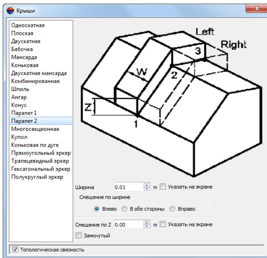
Рис. 51. Крыша типа «Парапет», где W — Ширина парапета, Z — высота парапета, Left и Right — расположение парапета, относительно сегментов полилинии (между вершинами 1, 2, 3 и далее), определяющей расположение парапета в плане ( Смещение по ширине ).
