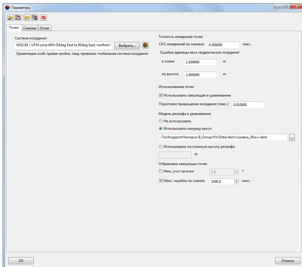
Рис. 23. Окно «Параметры»
