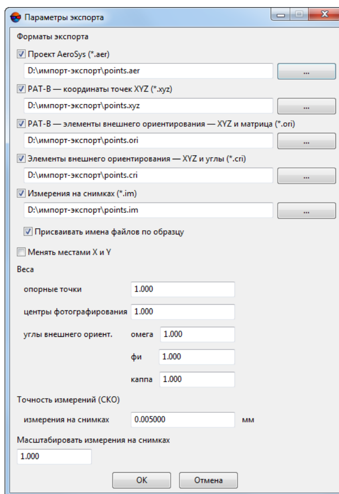
Рис. 45. Параметры экспорта
