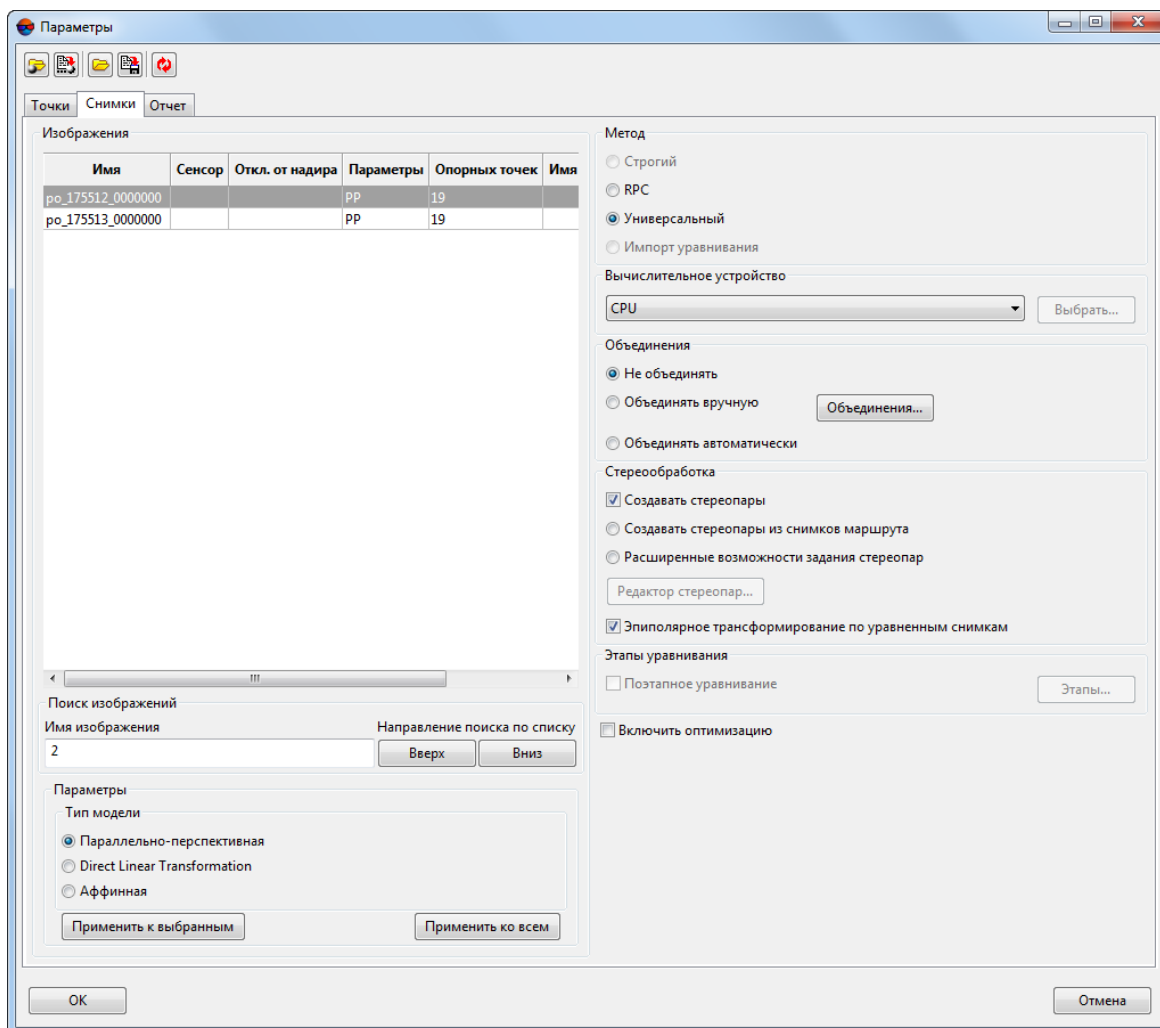
Рис. 25. Параметры уравнивания
