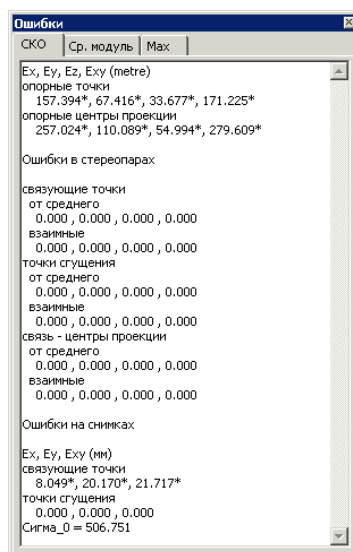
Рис. 8. Окно «Ошибки»
