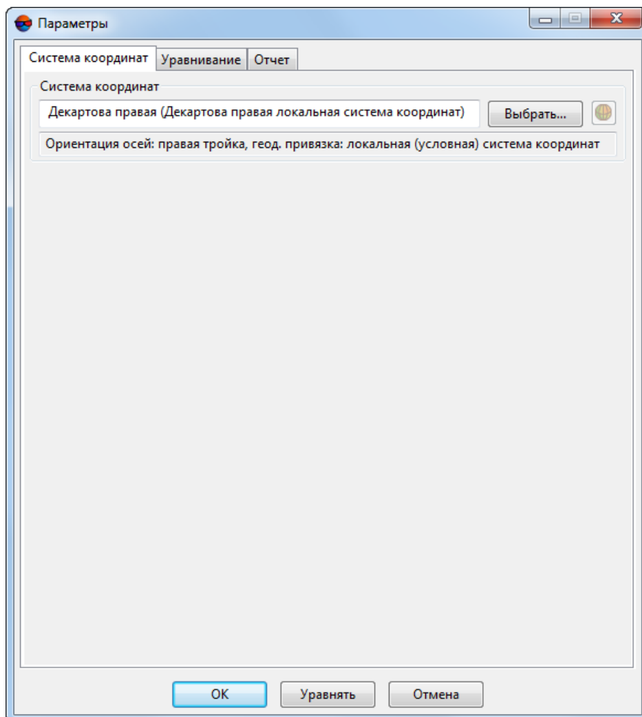
Рис. 10. Параметры уравнивания
