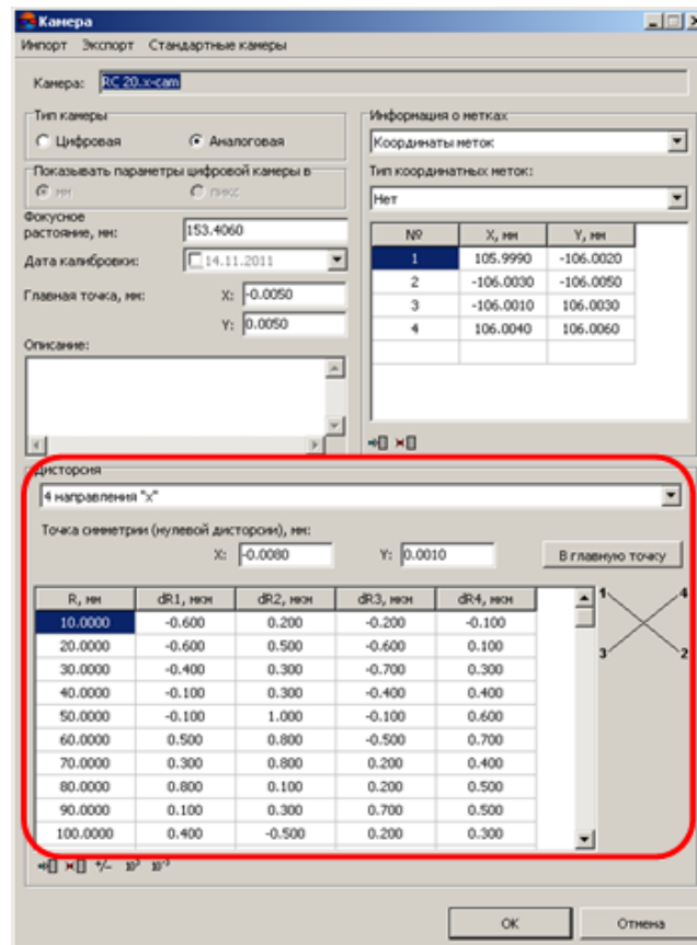
Рис. 18. Исходные табличные данные дисторсии из паспорта камеры, заданные в окне «Камера» на этапе ввода параметров камеры
