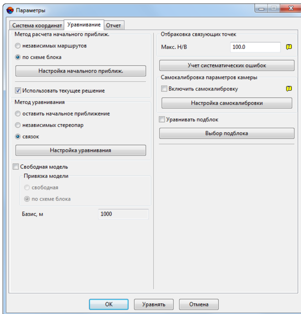
Рис. 11. Параметры уравнивания
