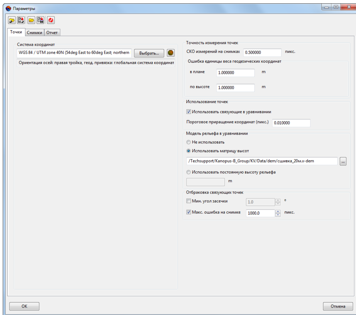
Рис. 24. Параметры уравнивания
