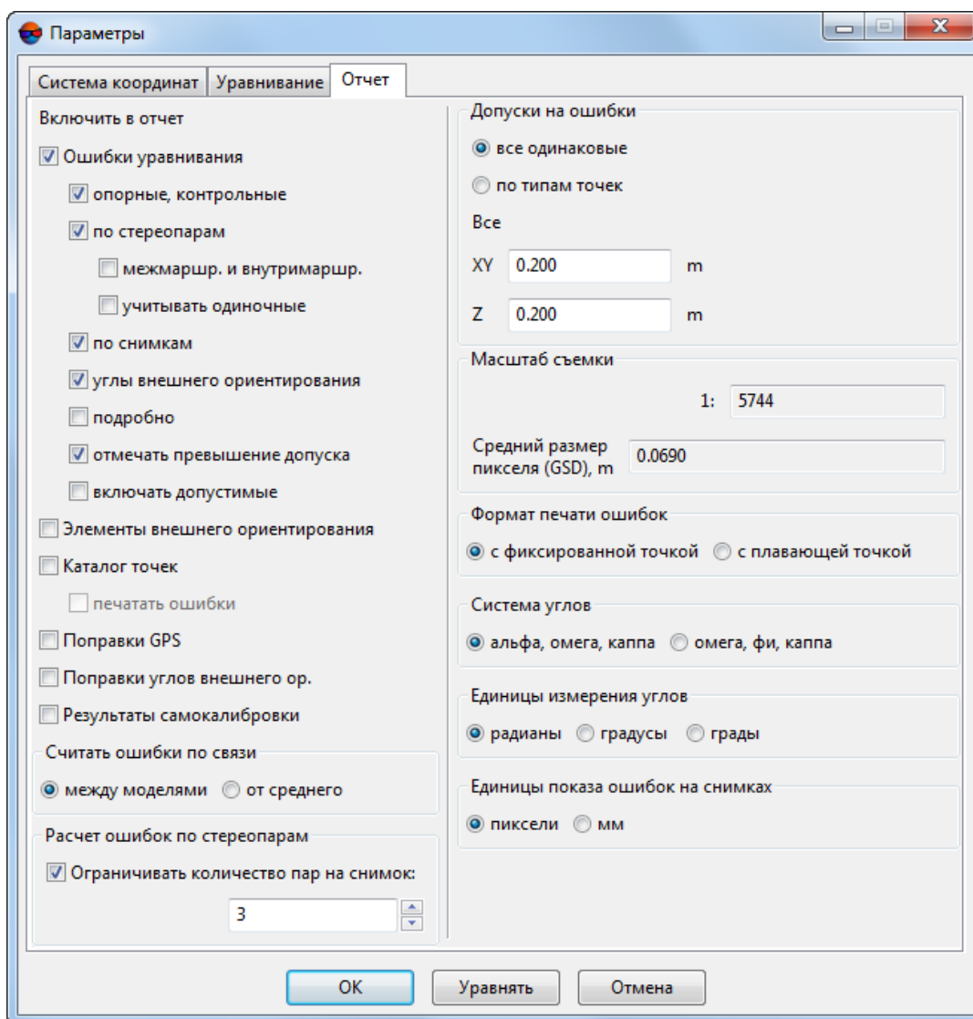
Рис. 22. Окно «Параметры»
