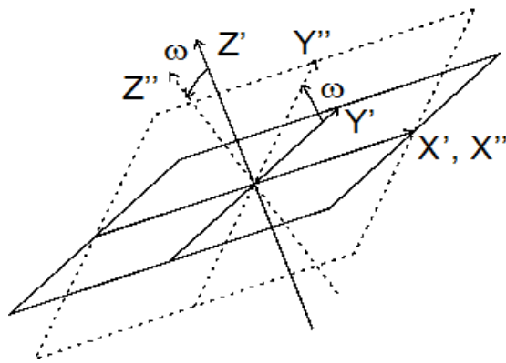
Рис. А.5. Положительный поворот вокруг оси X на угол «омега»
