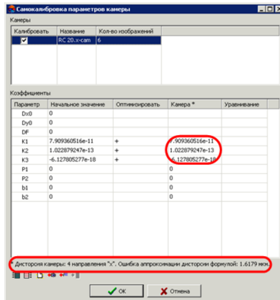
Рис. 19. Коэффициенты дисторсии K1, K2, K3, вычисленные в результате аппроксимации формулой, и ошибка дисторсии
