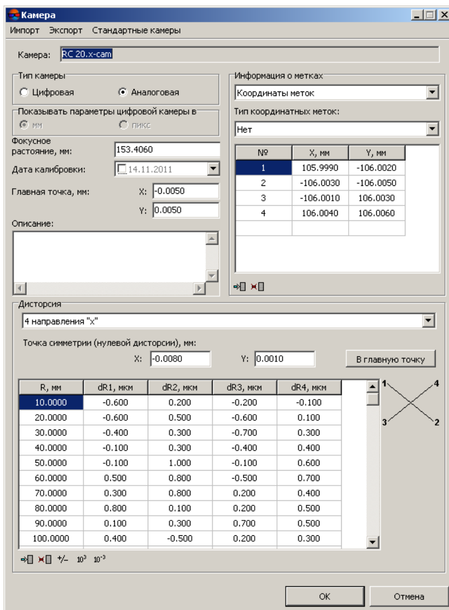
Рис. 9. Параметры аналоговой камеры
