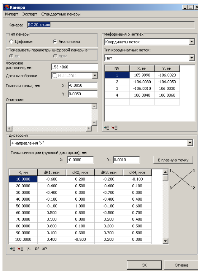
Рис. 10. Параметры аналоговой камеры
