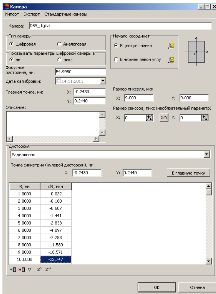
Рис. 15. Параметры цифровой камеры на примере камеры DSS
