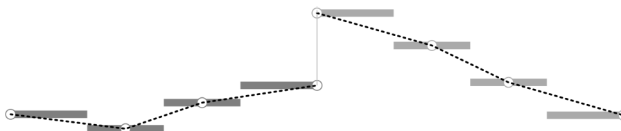
Рис. 23. 3D-модель, разбитая на тайлы, с границей тайла, проходящей по участку с сильно расчлененным рельефом (в центре)
