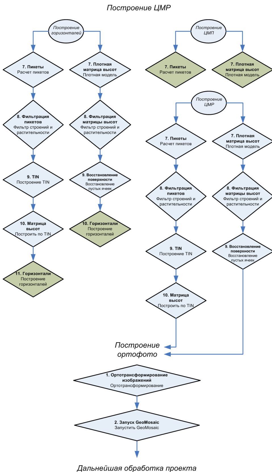
Рис. 13. Схема обработки проекта БПЛА (продолжение)
