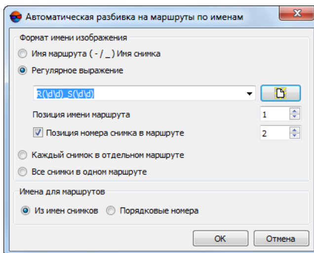
Рис. 48. Распределение на маршруты по именам изображений
