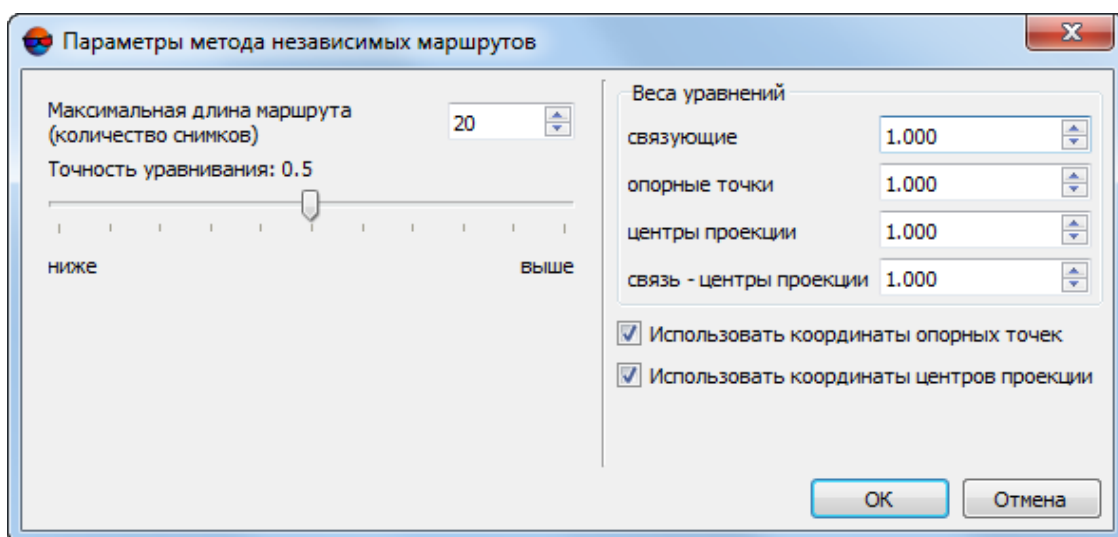
Рис. 13. Окно «Параметры метода независимых маршрутов»
