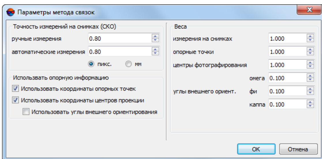
Рис. 16. Окно «Параметры метода связок»
