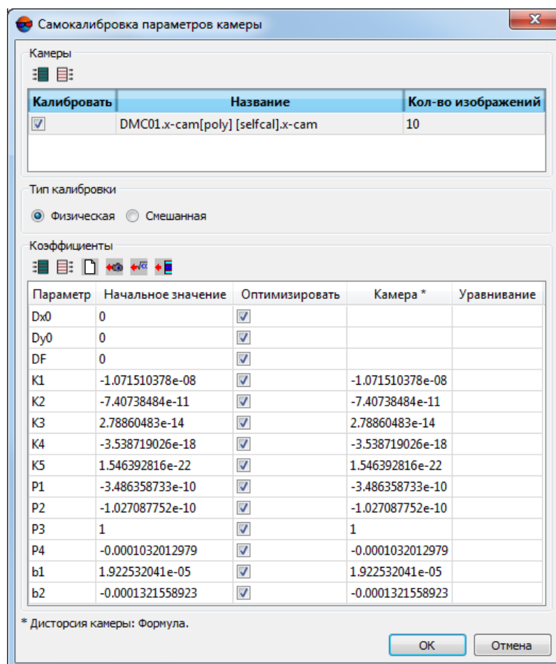
Рис. 17. Окно «Самокалибровка параметров камеры»
