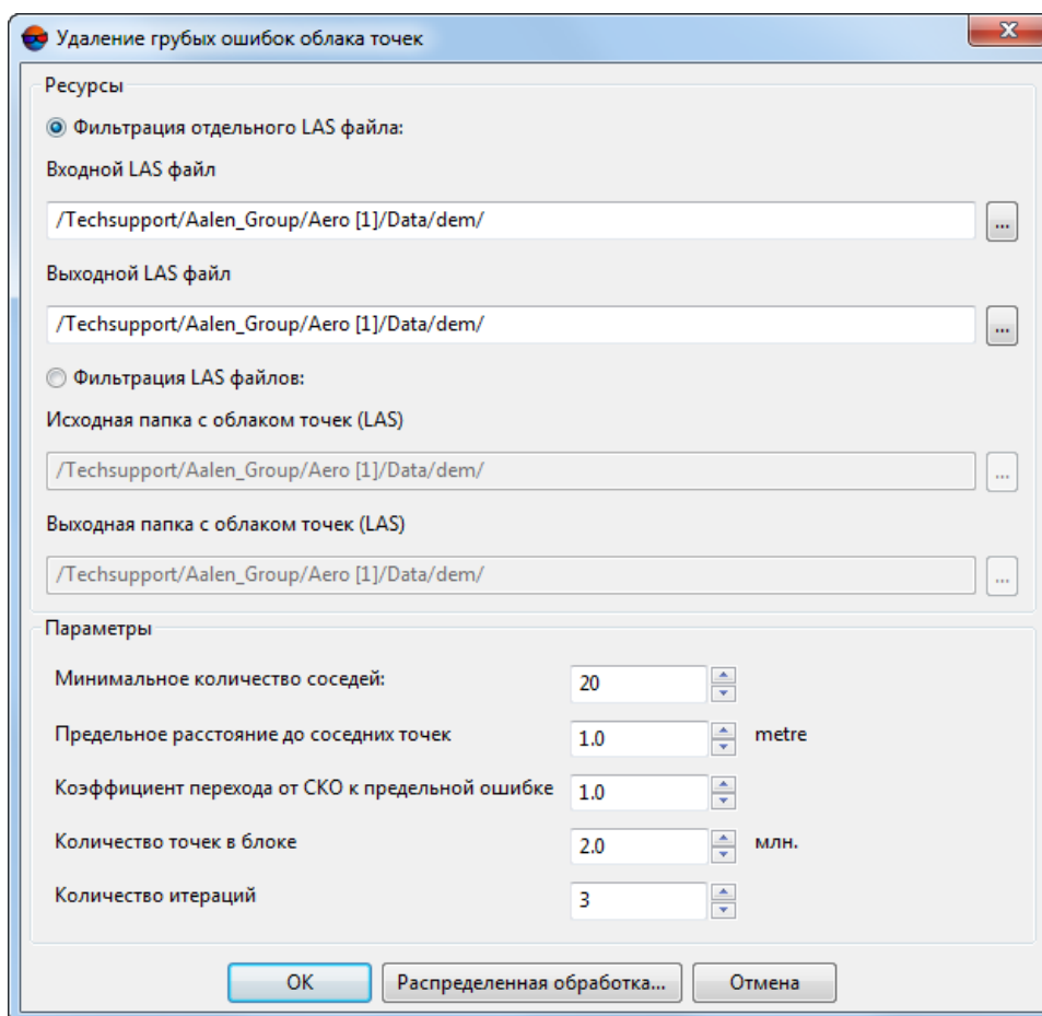
Рис. 33. Окно «Удаление грубых ошибок облака точек»
