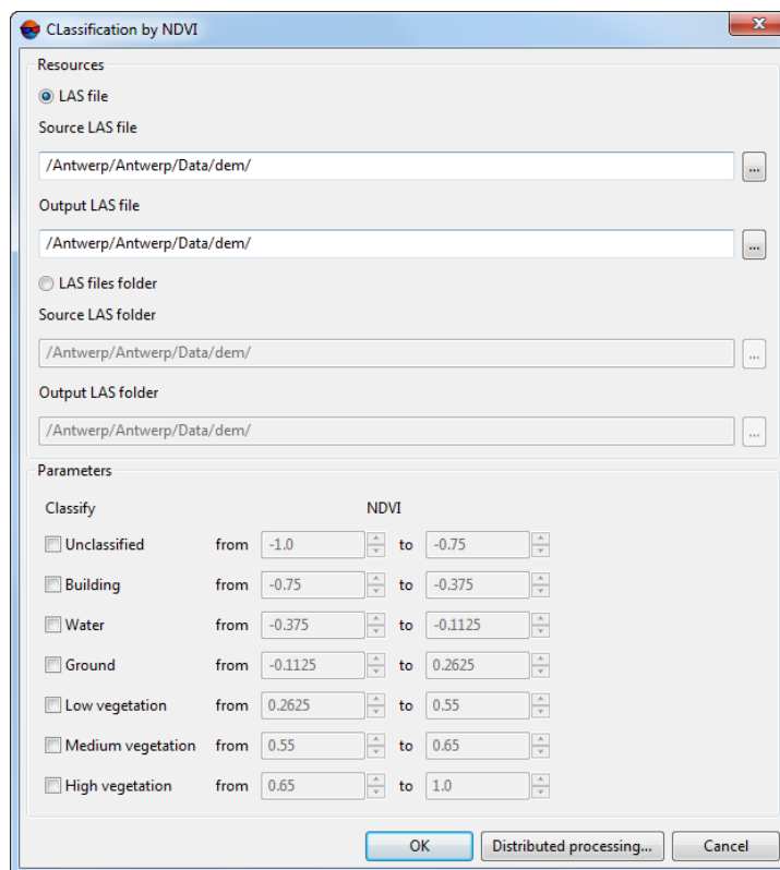
Рис. 25. Окно «Классификация по NDVI»
