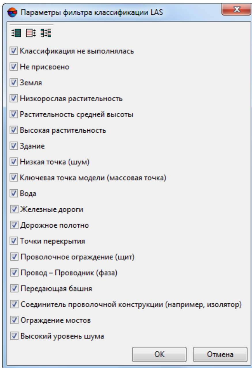
Рис. 13. Окно «Параметры фильтра классификации LAS»
