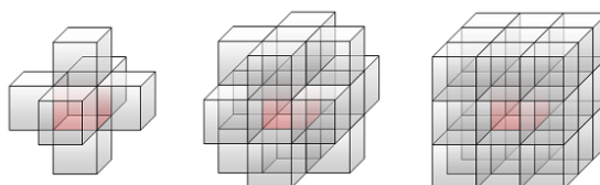
Рис. 22. Обрабатываемый воксель (выделен красным) и ближайшие соседние 6, 18 или 26 вокселей
