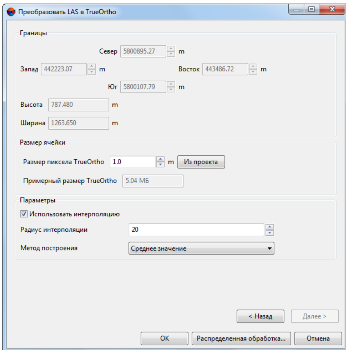
Рис. 16. Окно «Преобразовать LAS в True Ortho»
