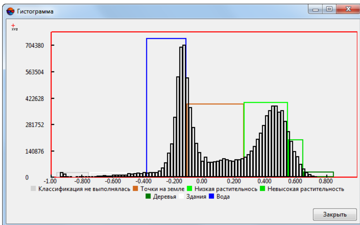
Рис. 28. Окно «Гистограмма»
