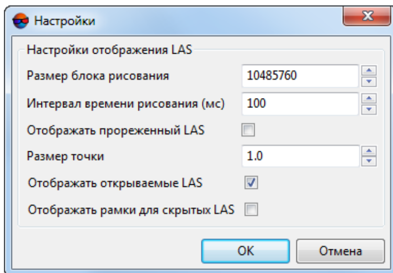
Рис. 3. Окно «Настройки»
