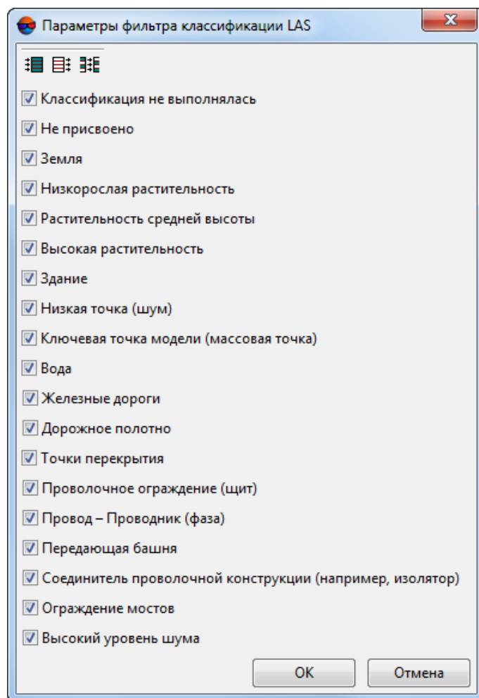
Рис. 30. Окно «Параметры фильтра классификации LAS»
