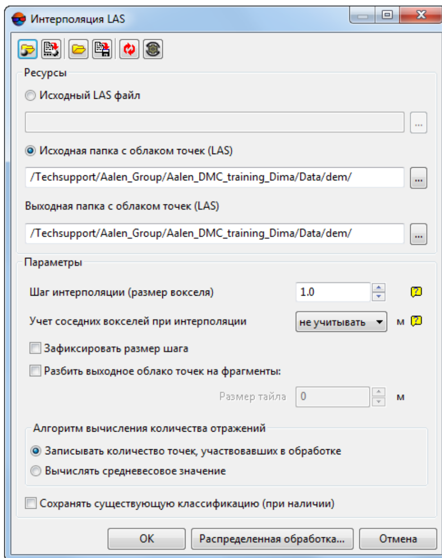
Рис. 21. Окно «Интерполяция LAS»
