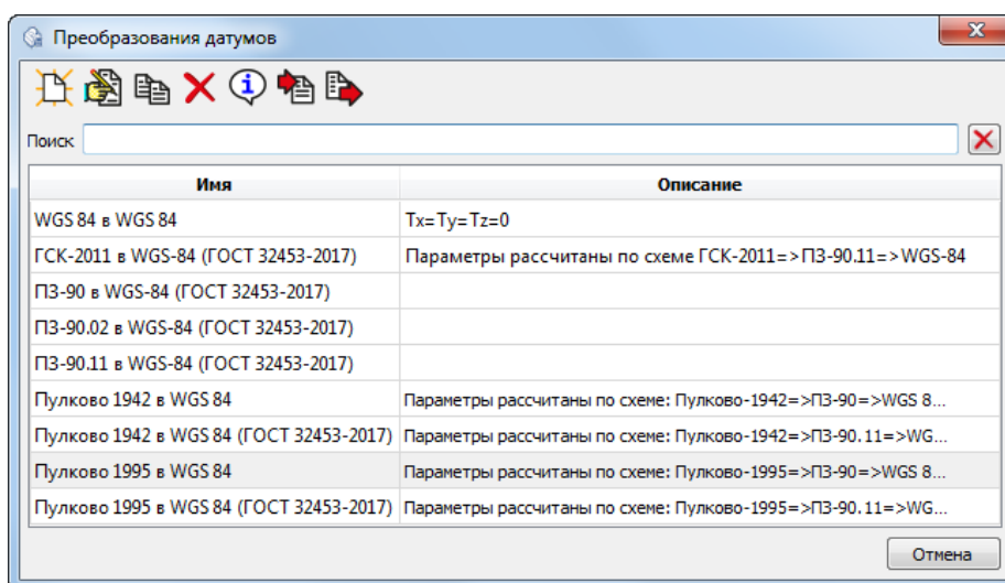
Рис. 16. Стандартные наборы параметров преобразования датумов
