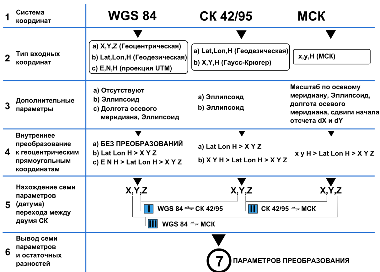
Рис. Е.17. Схема вычисления параметров преобразования между двумя системами координат
