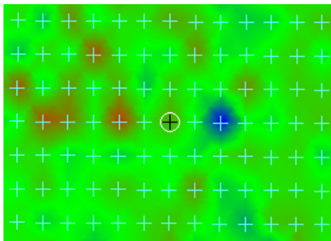
Рис. 8. Выбор креста
