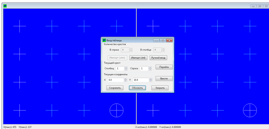
Рис. 20. Таблица крестов
