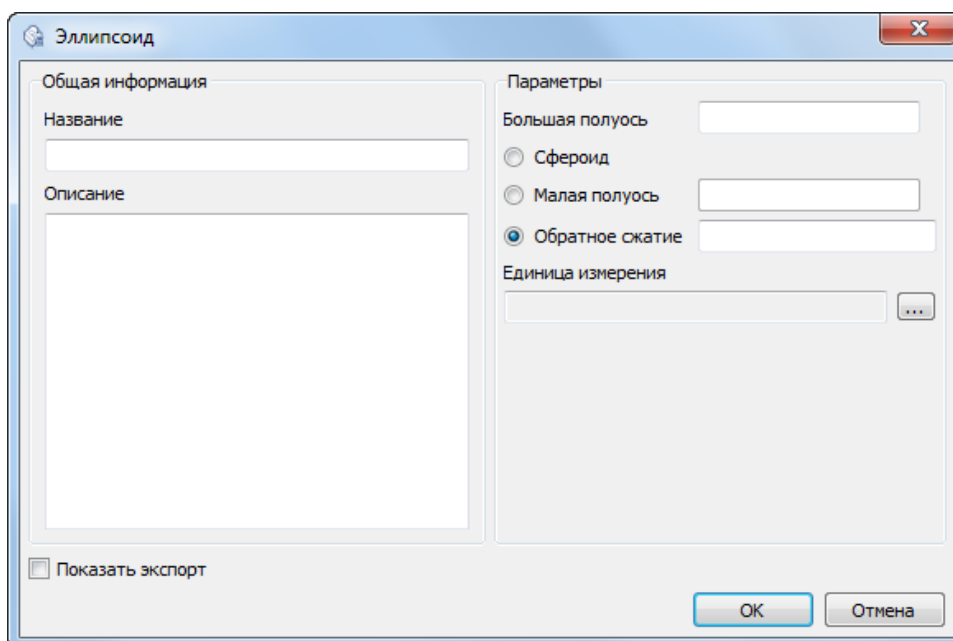
Рис. 27. Параметры референц-эллипсоида
