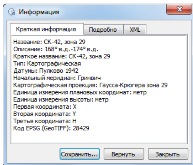
Рис. 6. Окно «Информация»
